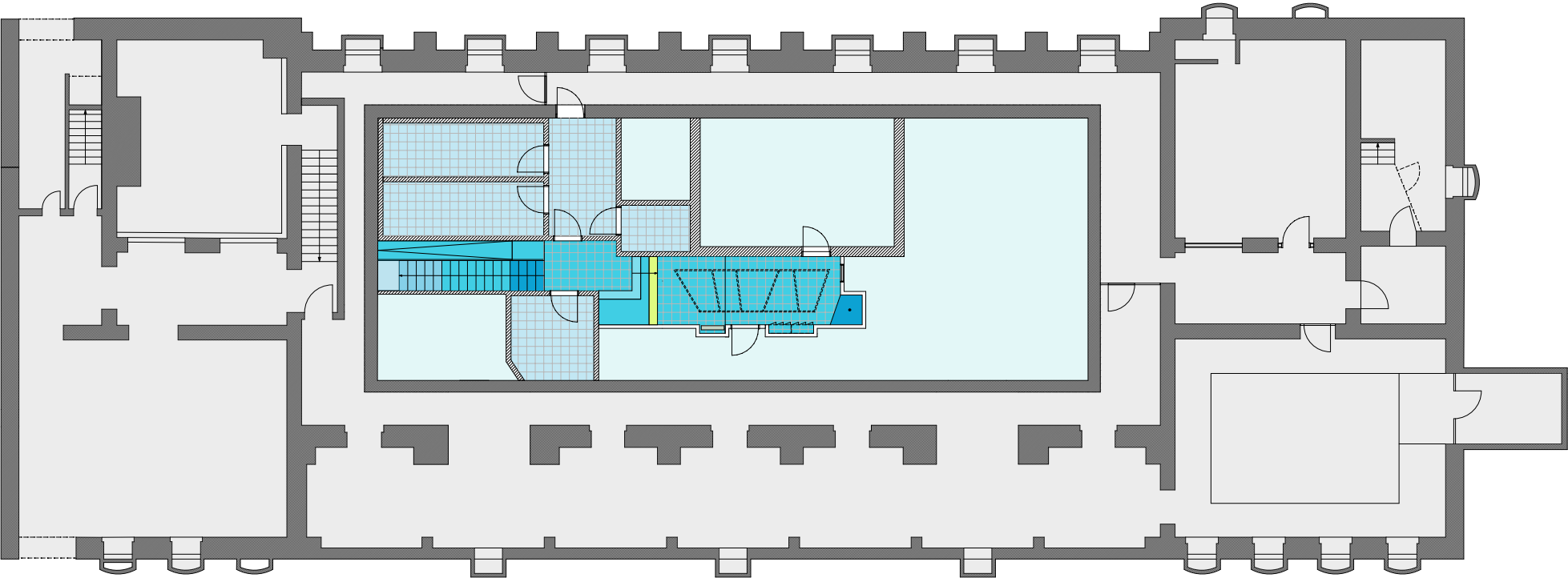
Grundriss KG
