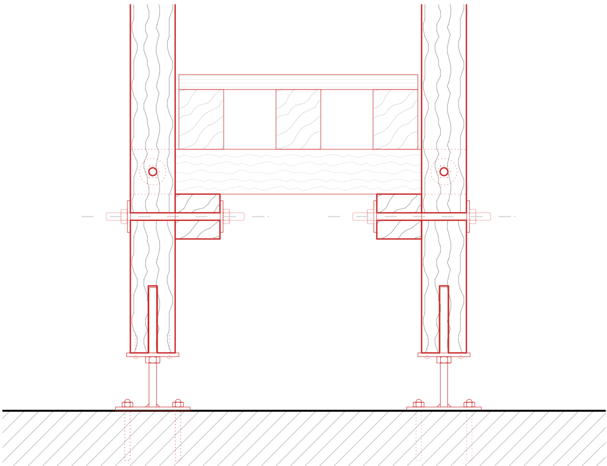
VERTIKALSCHNITT ECKSTÜTZE
