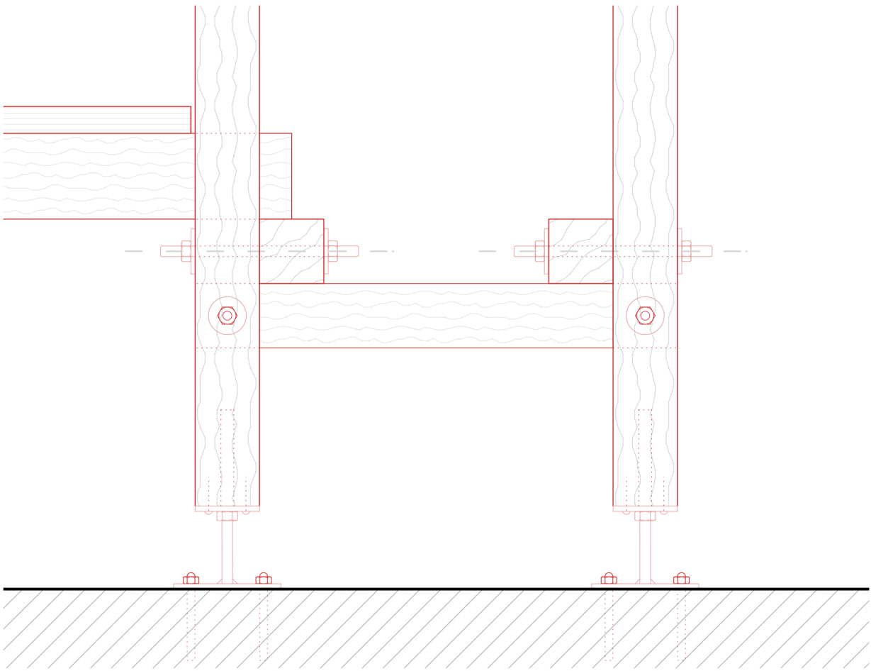
ANSICHT ECKSTÜTZE
