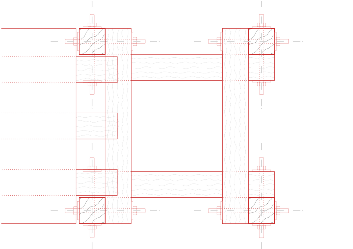
HORIZONTALSCHNITT ECKSTÜTZE
