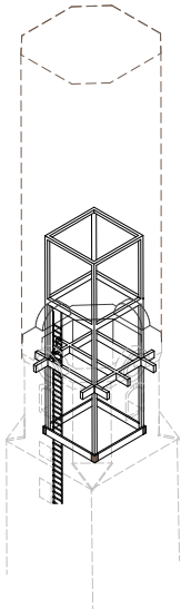
Konstruktion mit Schwingungsdämpfer
