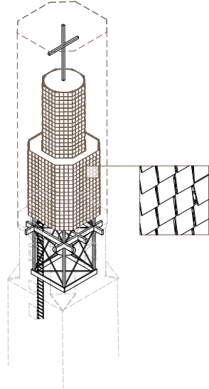
Fassadenelemente
