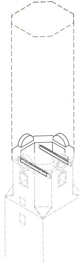
Konstruktion der Fassadenelemente
