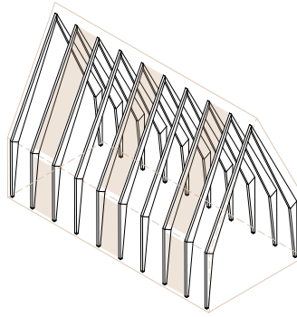
Konstruktion Holzstützen aus Baubuche oder Brettschichtholz
