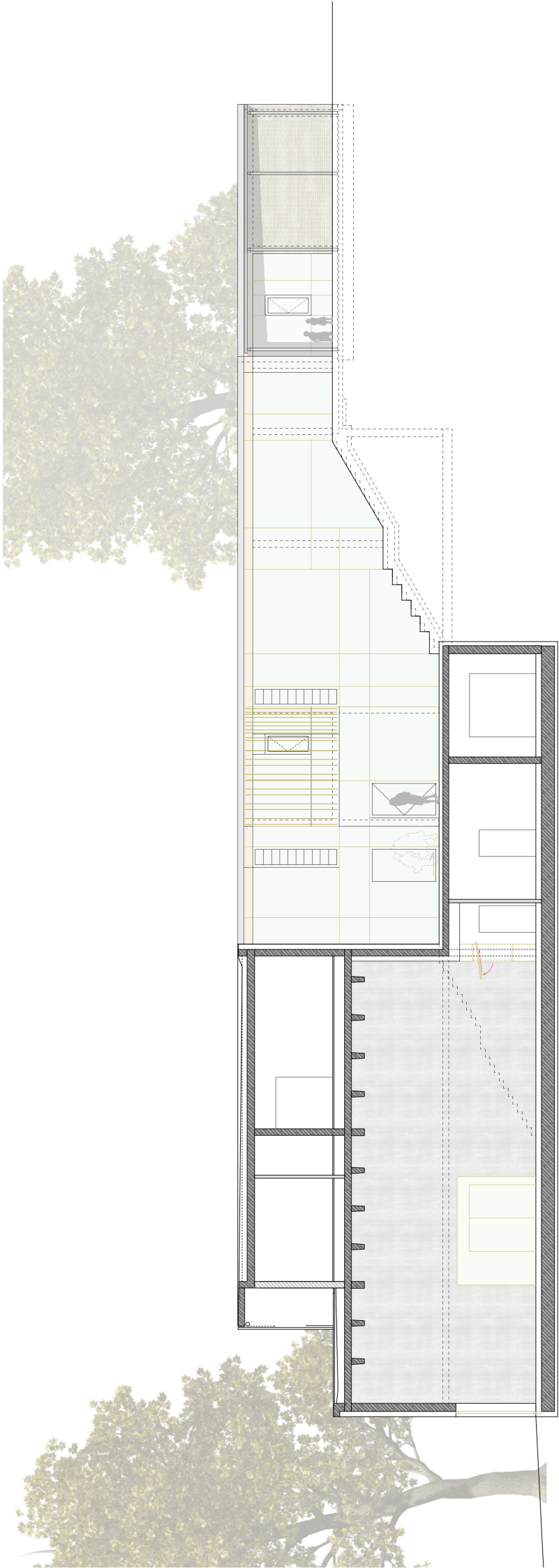
Schnitt E-E
