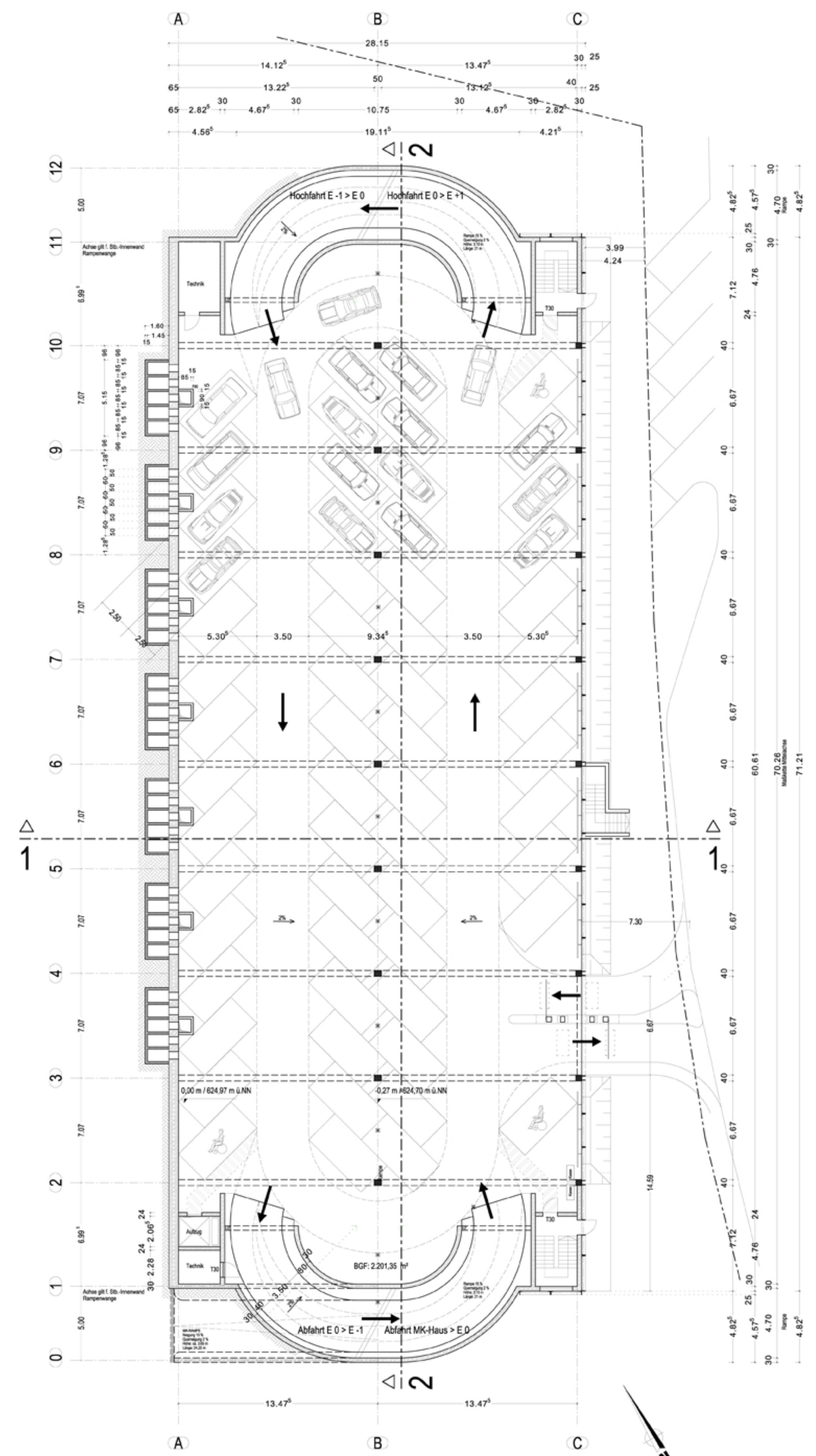
EBENE 0 / 624.97 m ü.NN / 59 Stpl. [M=1:200]
