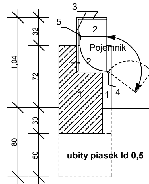
PRZEKROJ
