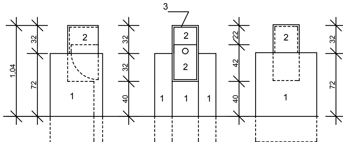
WIDOK 1+ 2+ 3
