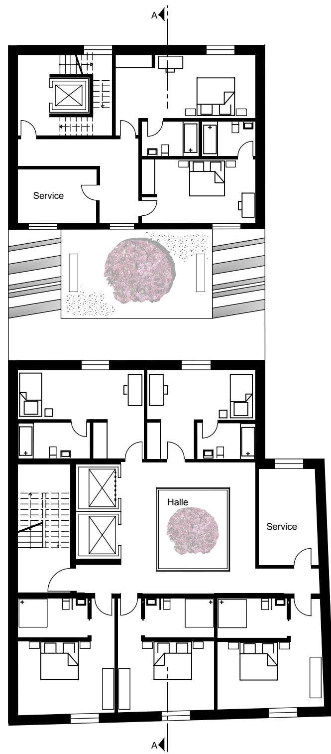
1. Obergeschoss
