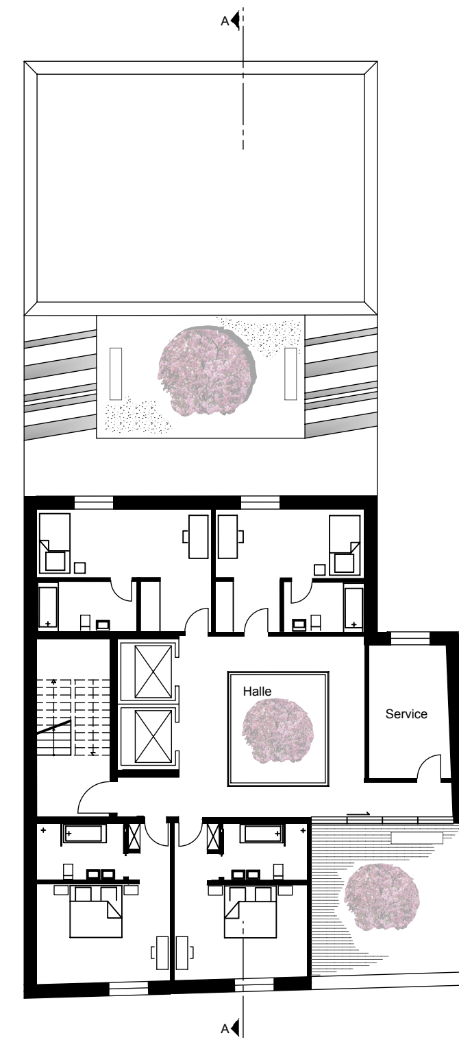
4. Obergeschoss
