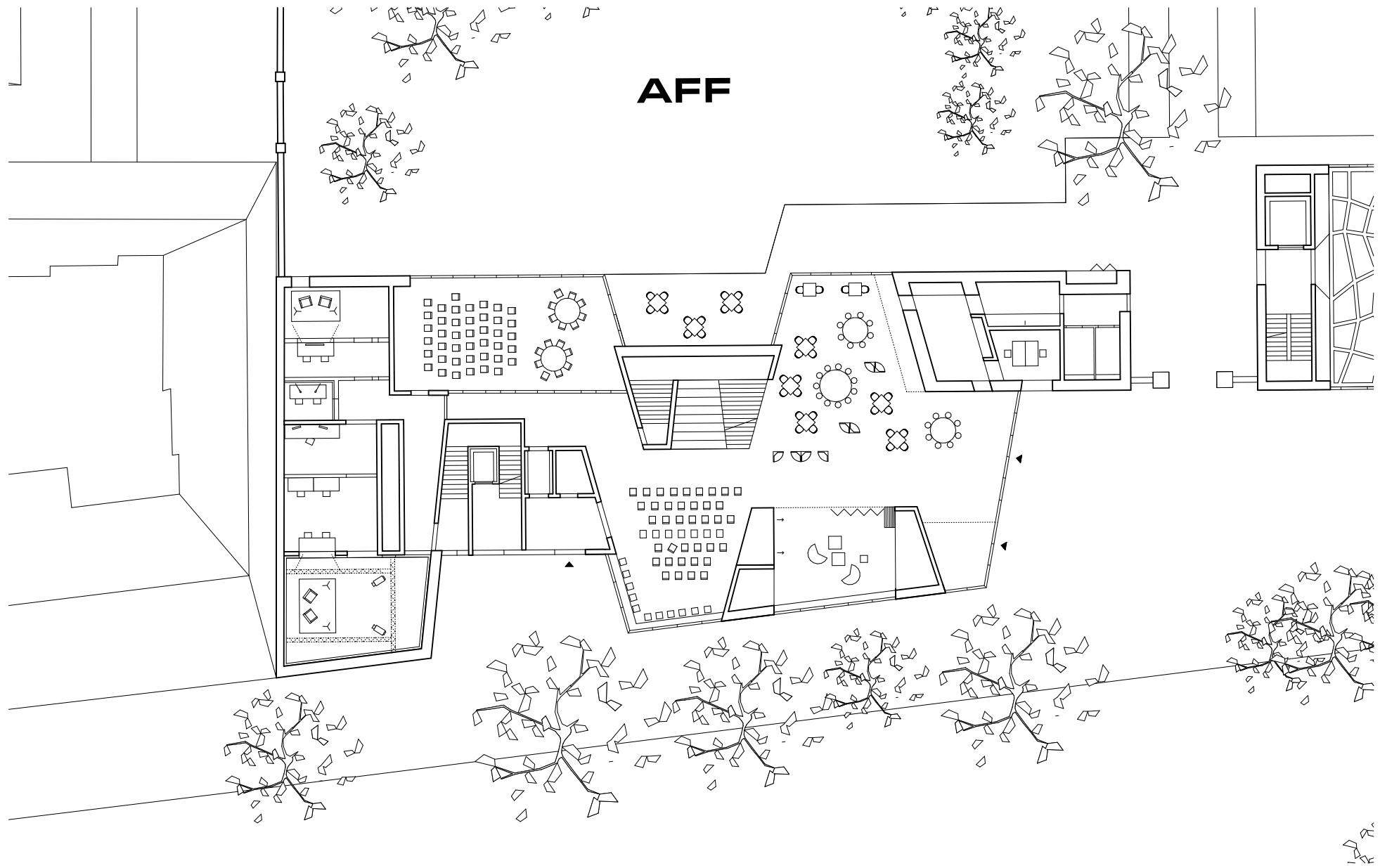
PUBLIX Grundriss Erdgeschoss - möbliert -
