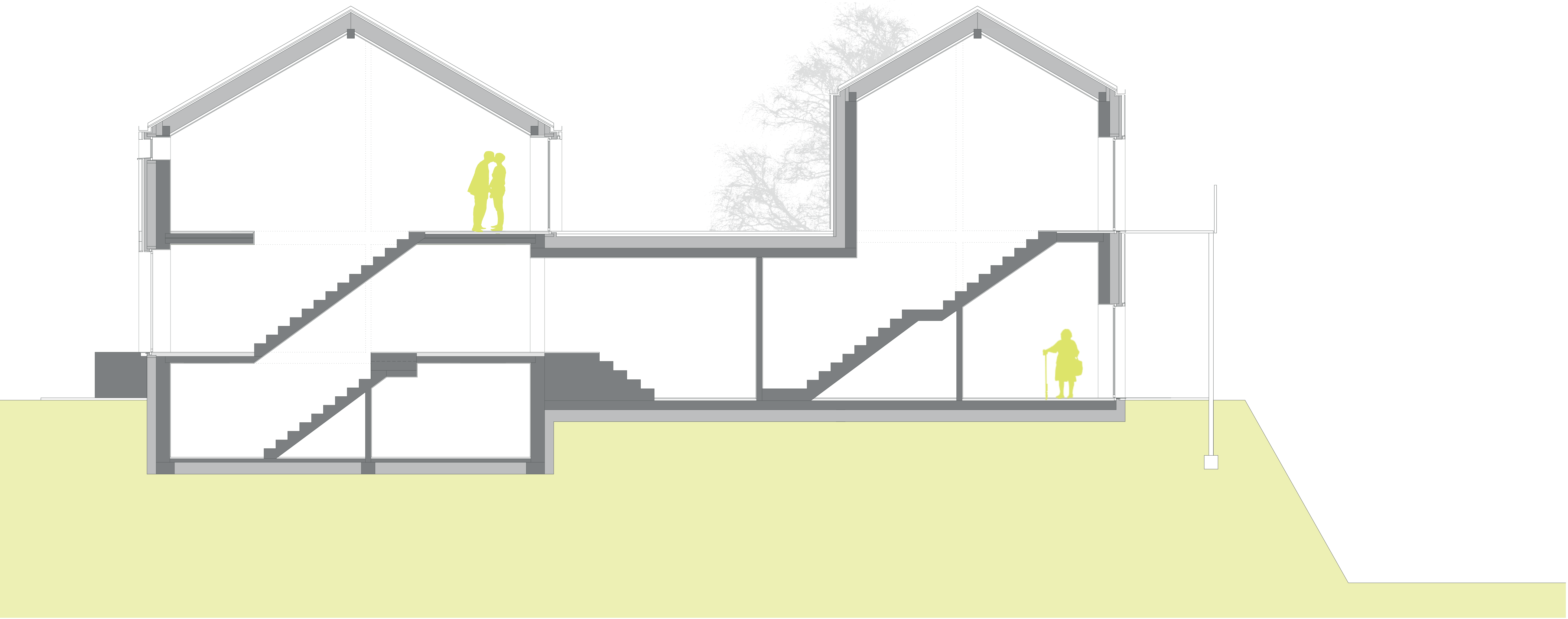
Schnitt
