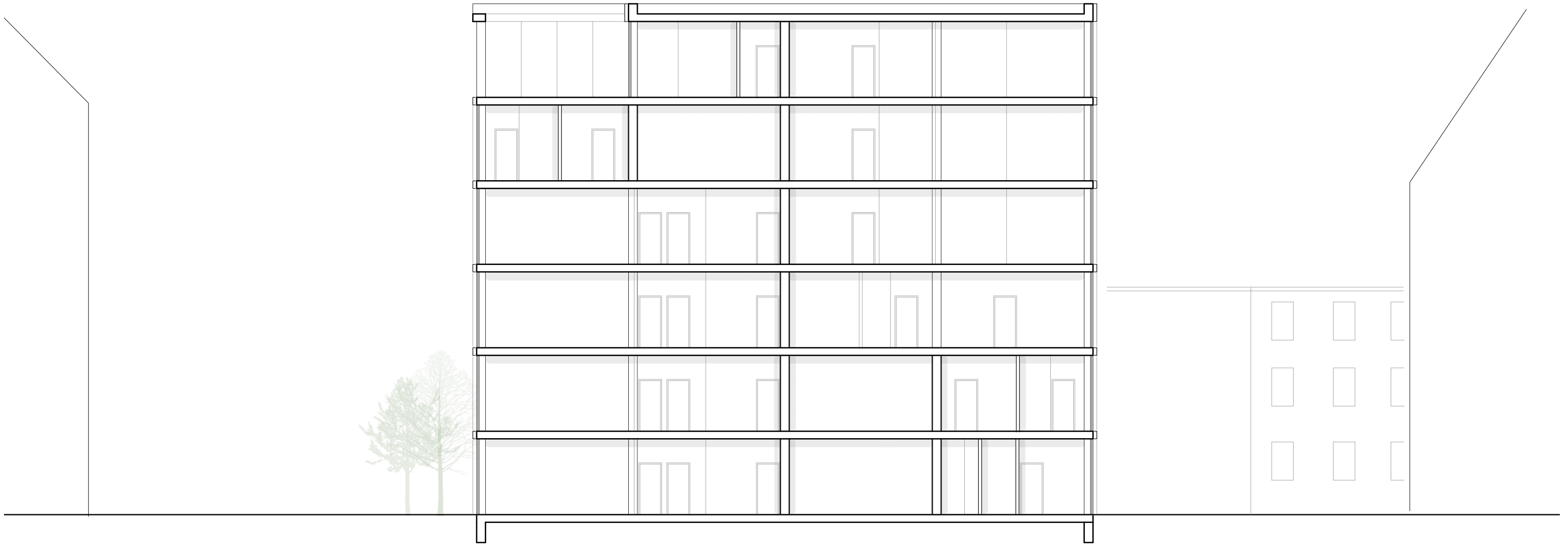
SCHNITT A : A M 1:150
