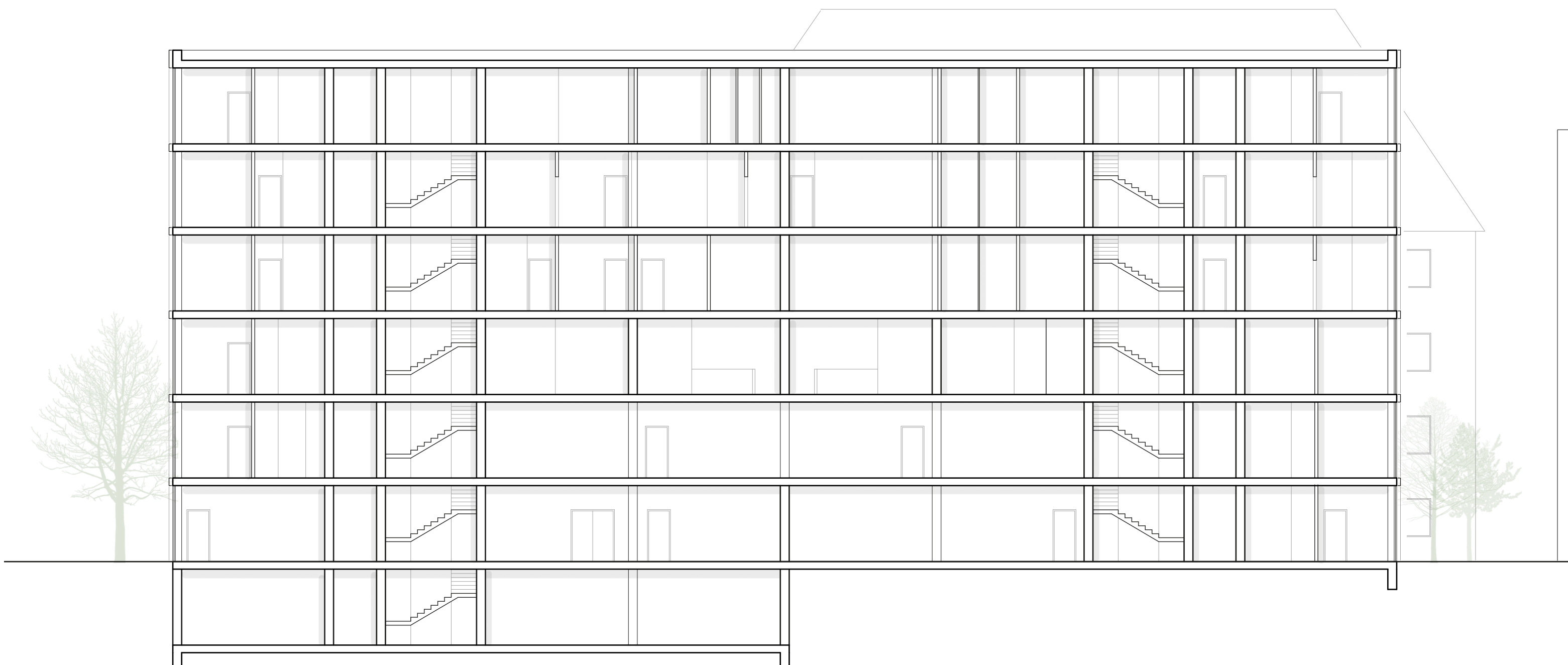
SCHNITT C : C M 1:150
