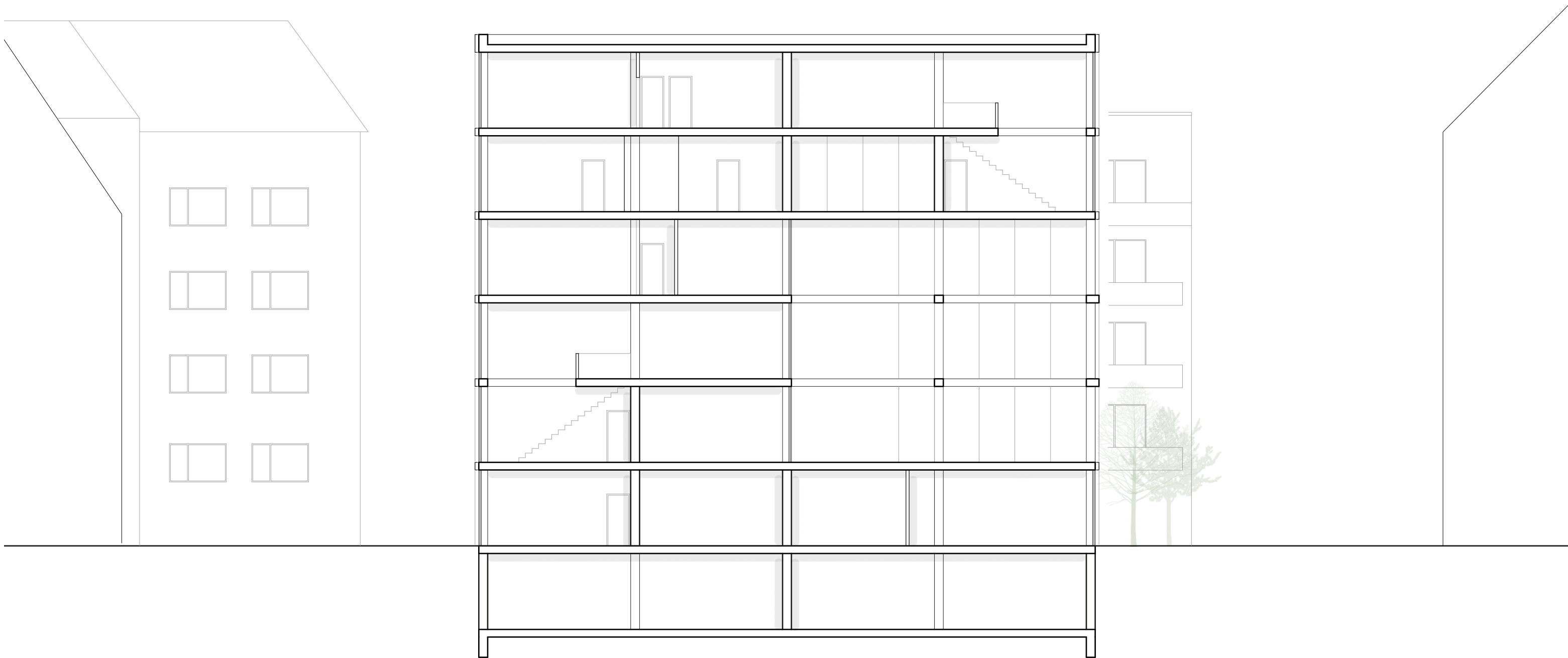
SCHNITT B : B M 1:150
