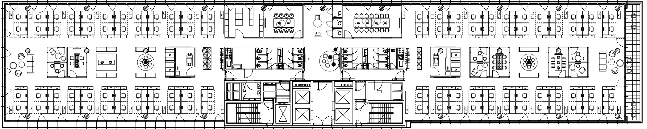
GR 15. Obergeschoss
