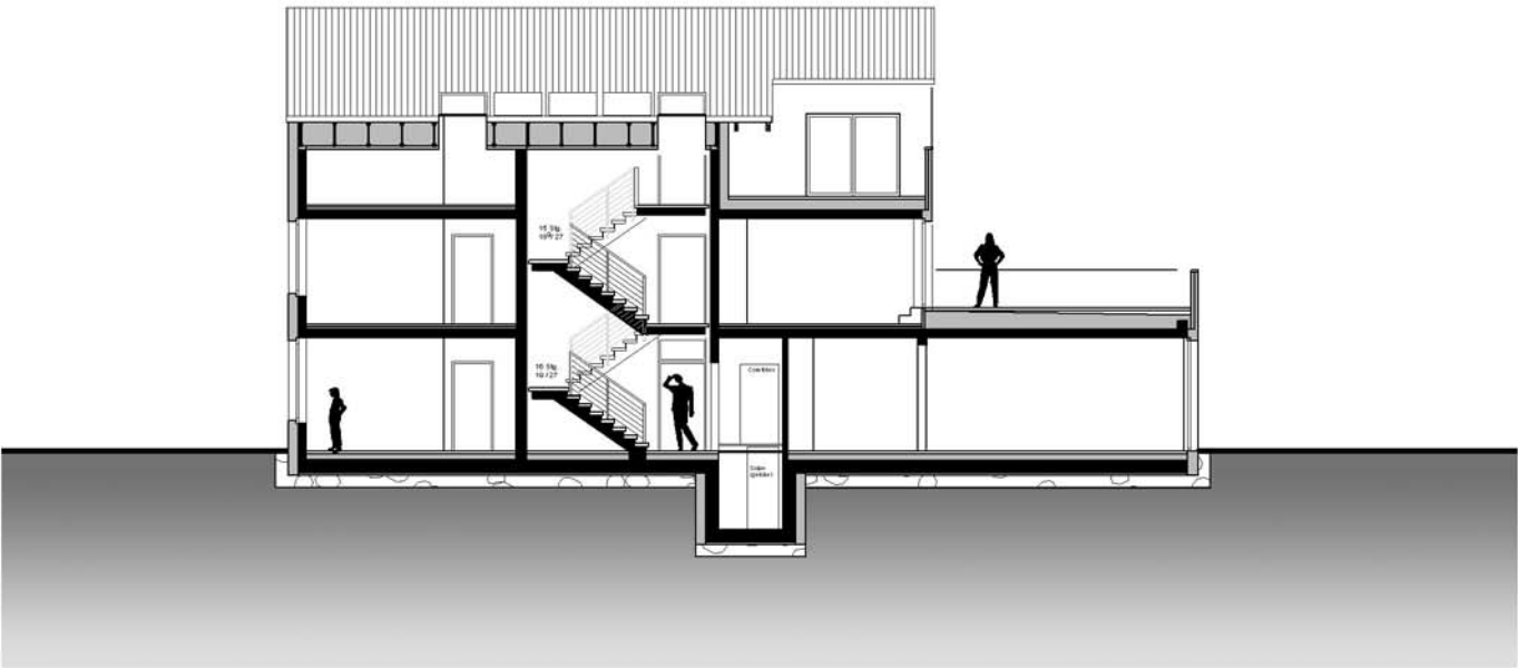
Schnitt A M 1:200
