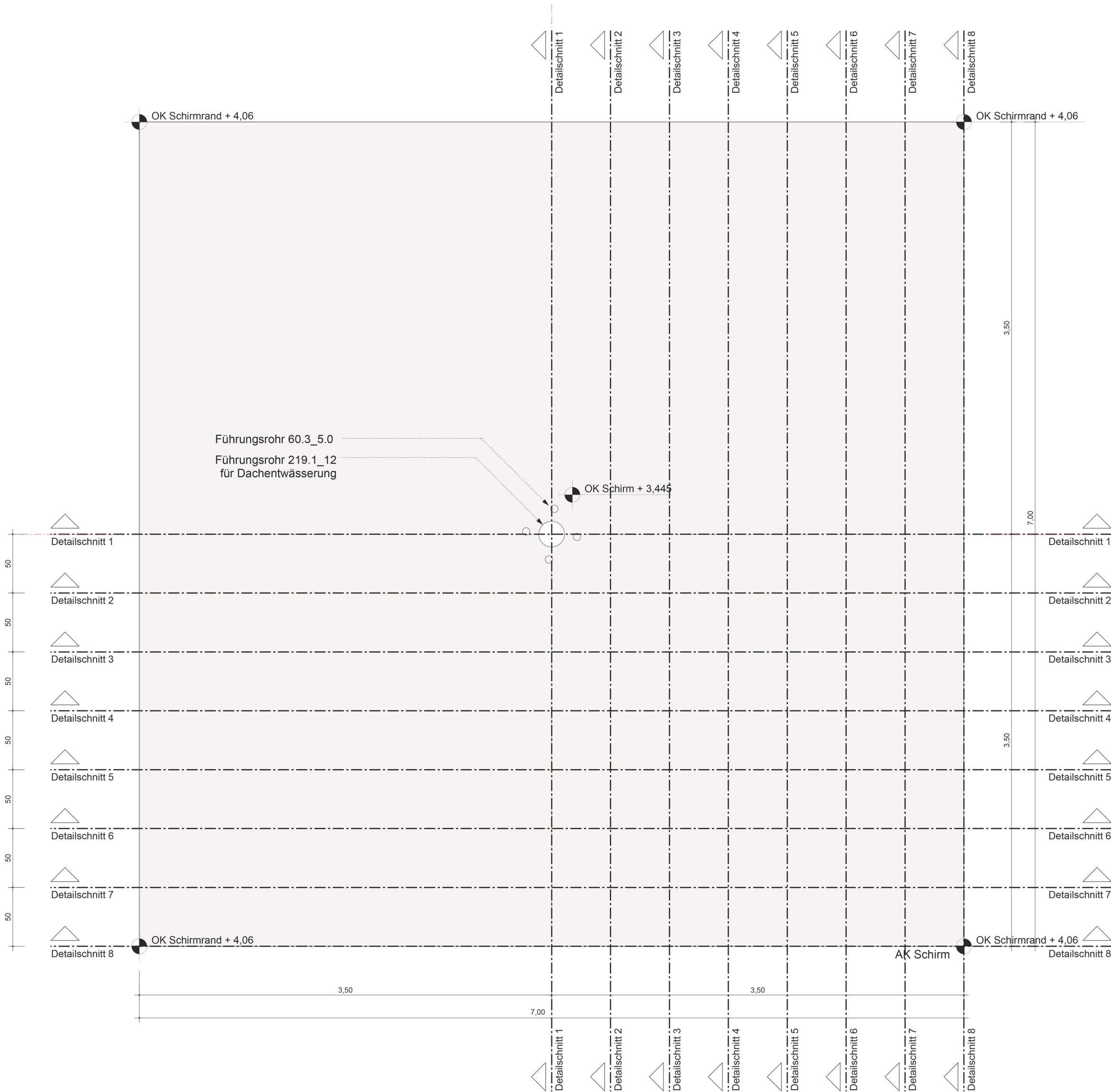
Prinzip Schalungsbau o.M.
