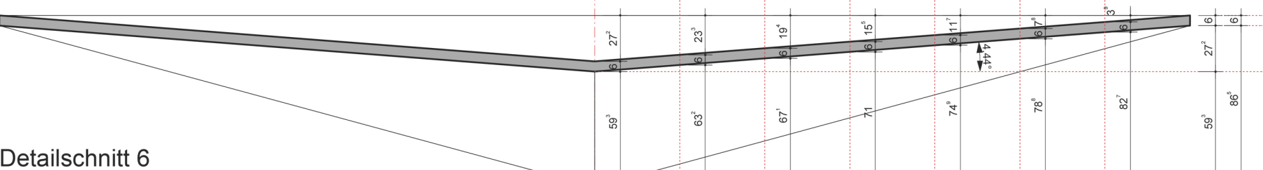
Detailschnitt 6
