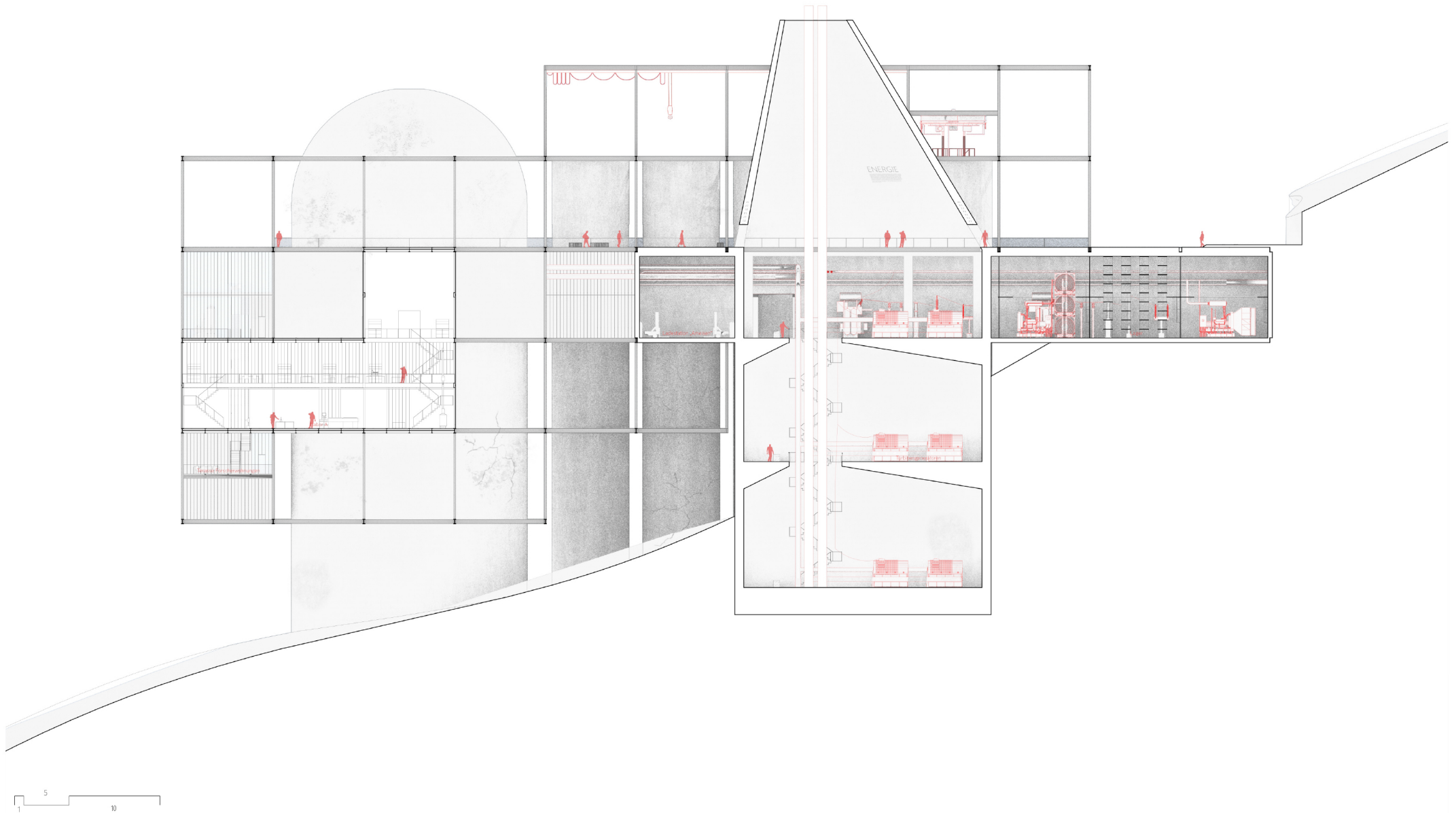
Schnitt N Kloster der Energien
