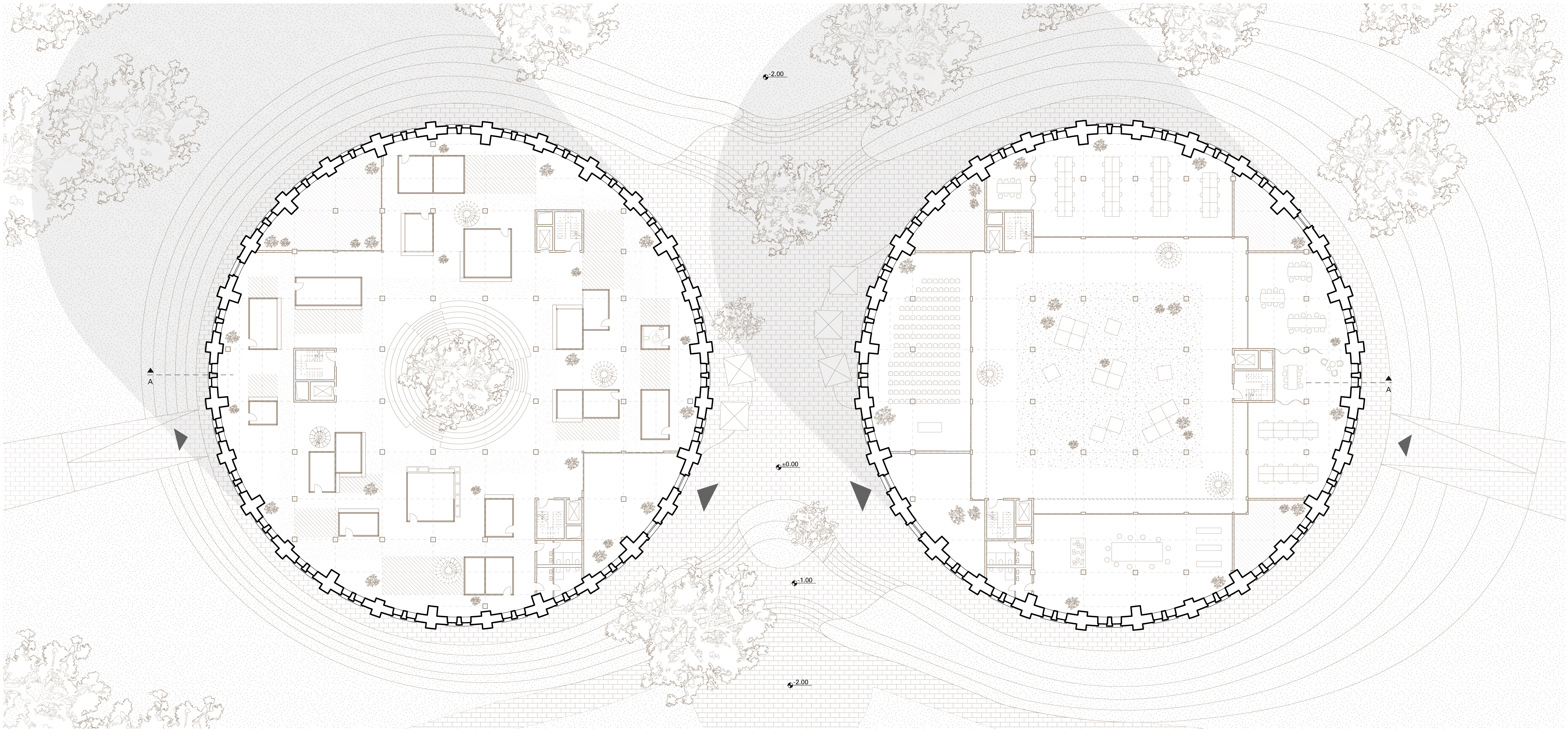
Grundriss Erdgeschoss 1:200
