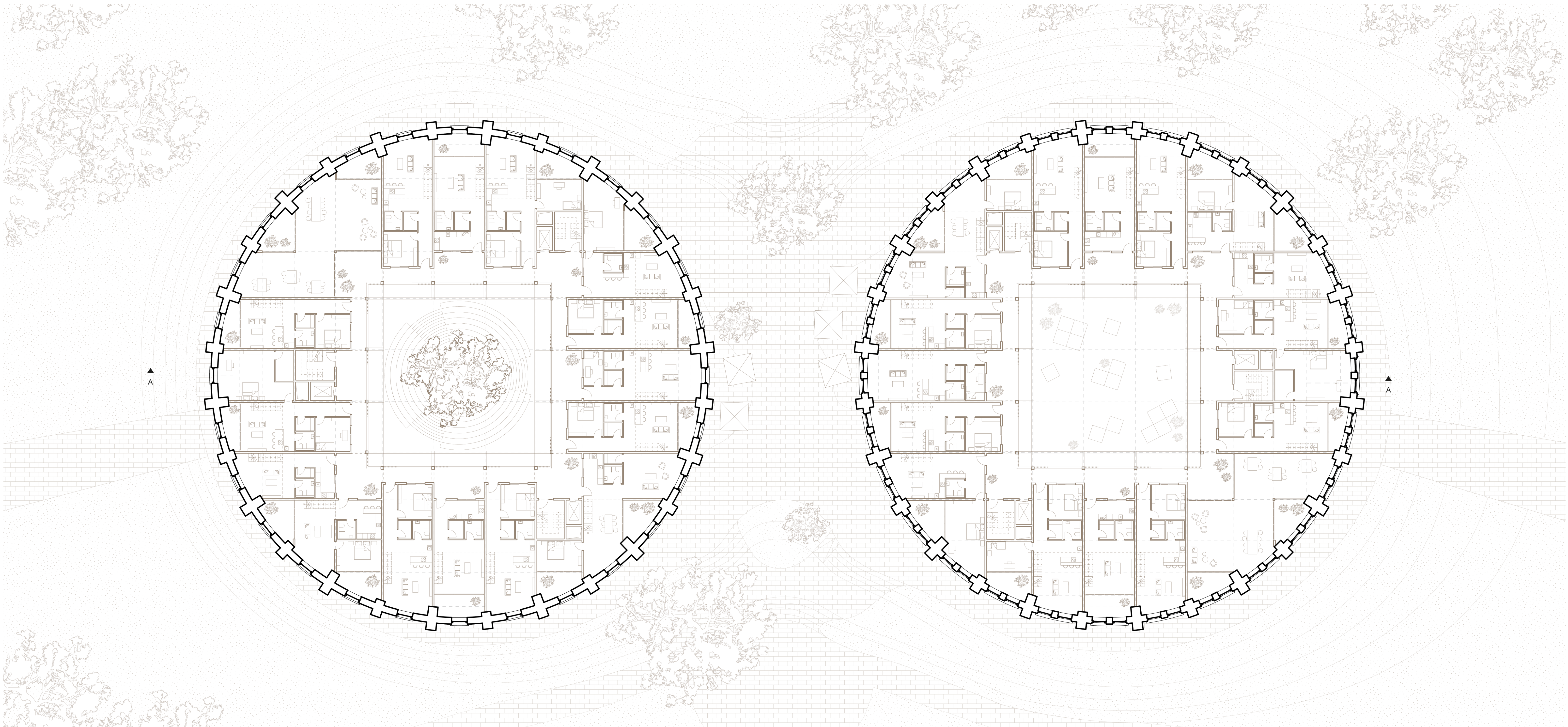
Grundriss Obergeschoss 1:200
