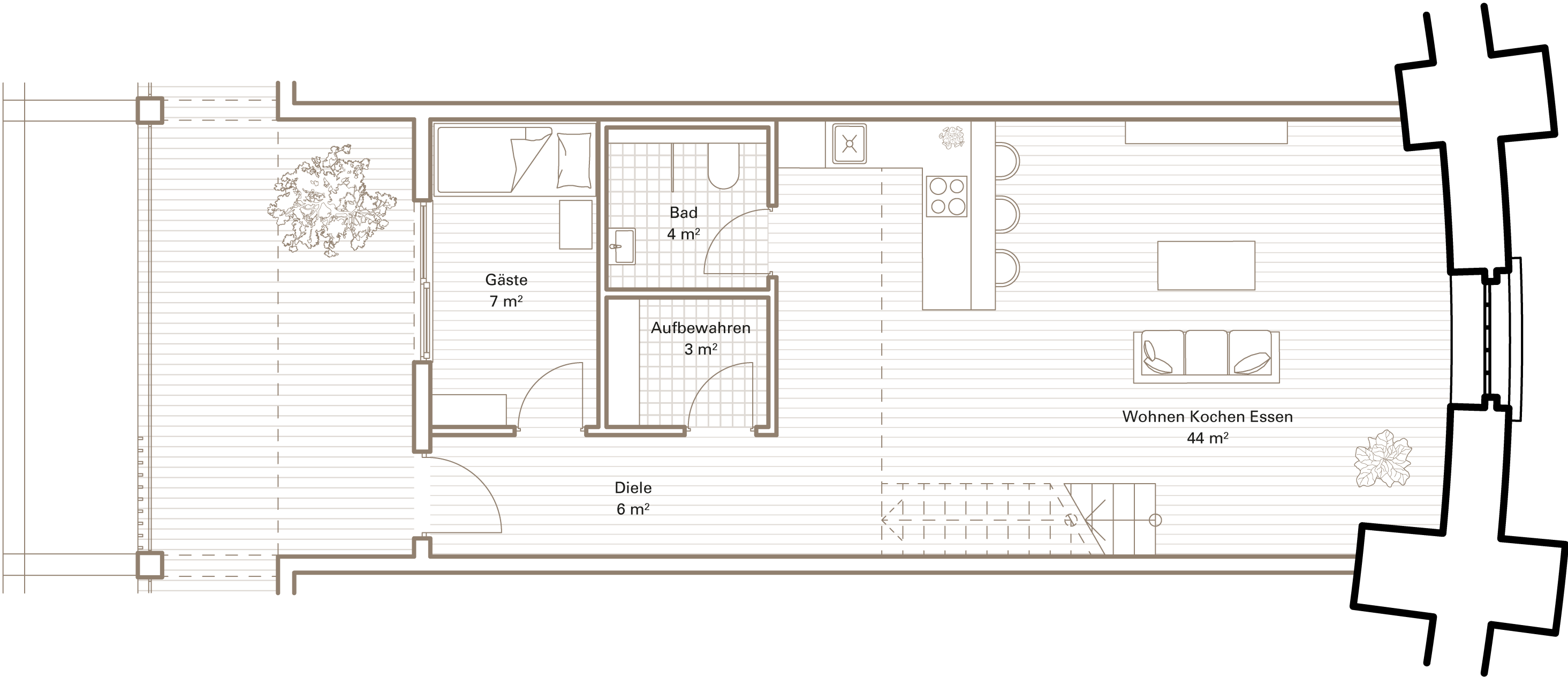
Grundriss Maisonettewohnung EG 1:50
