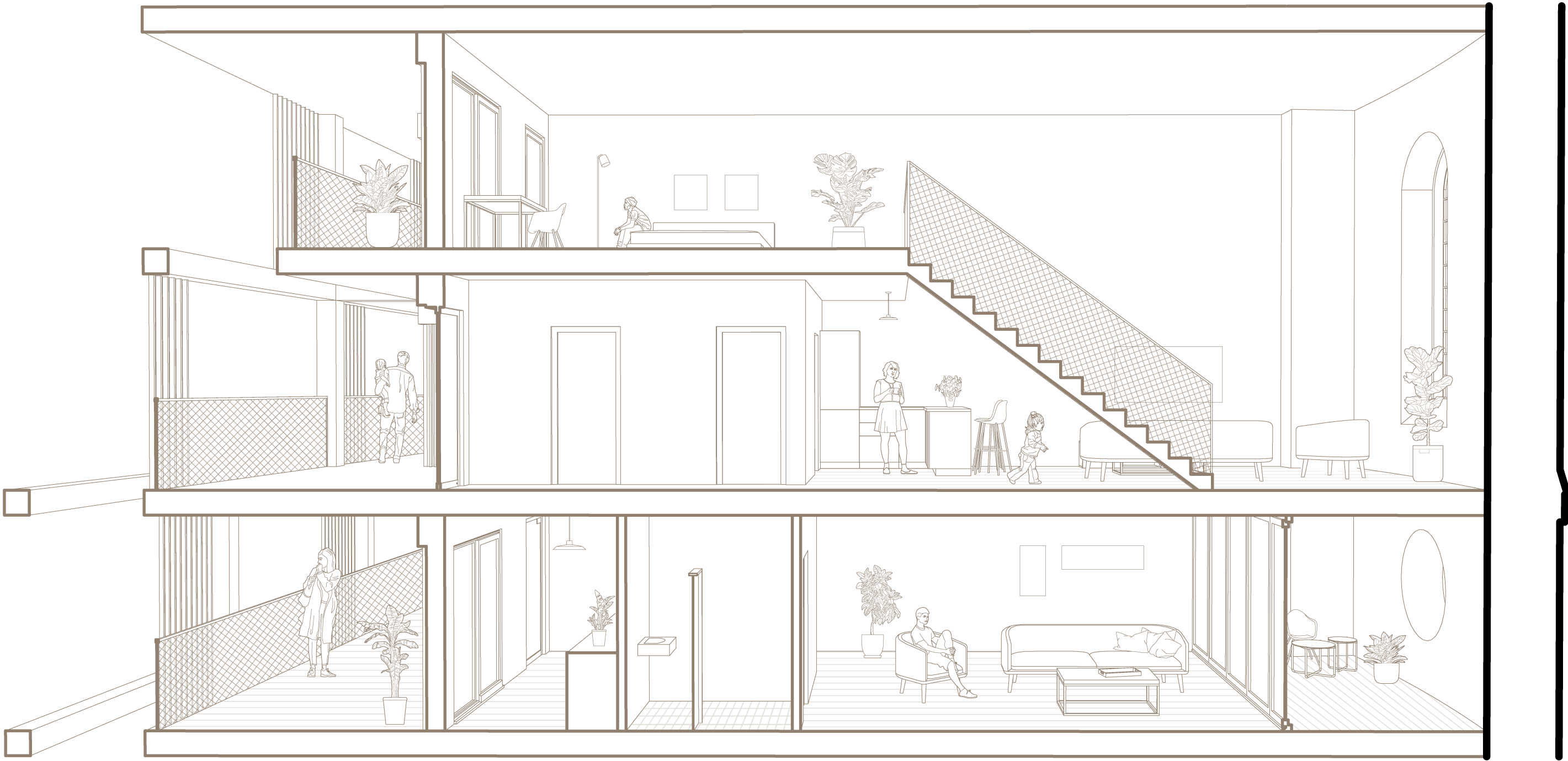
Schnitt Wohnungen
