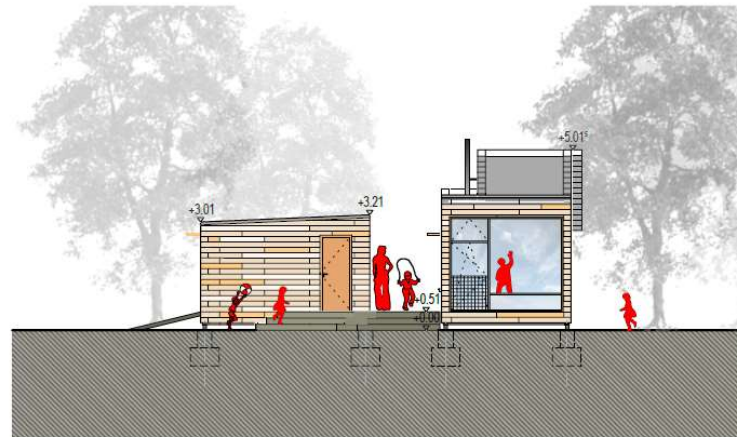
Ansicht Ost M1/100
