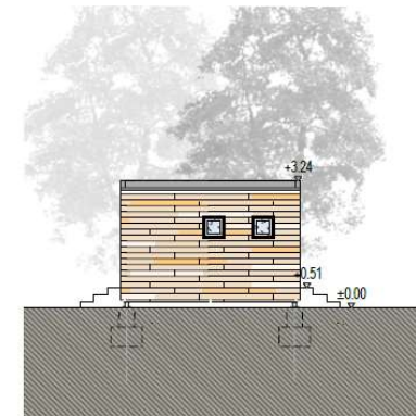
Ansicht Süd Gerätehütte M1/100
