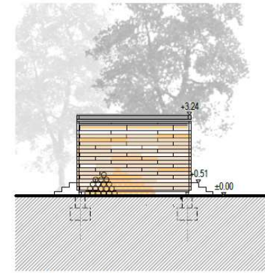
Ansicht Nord Gerätehütte M1/100
