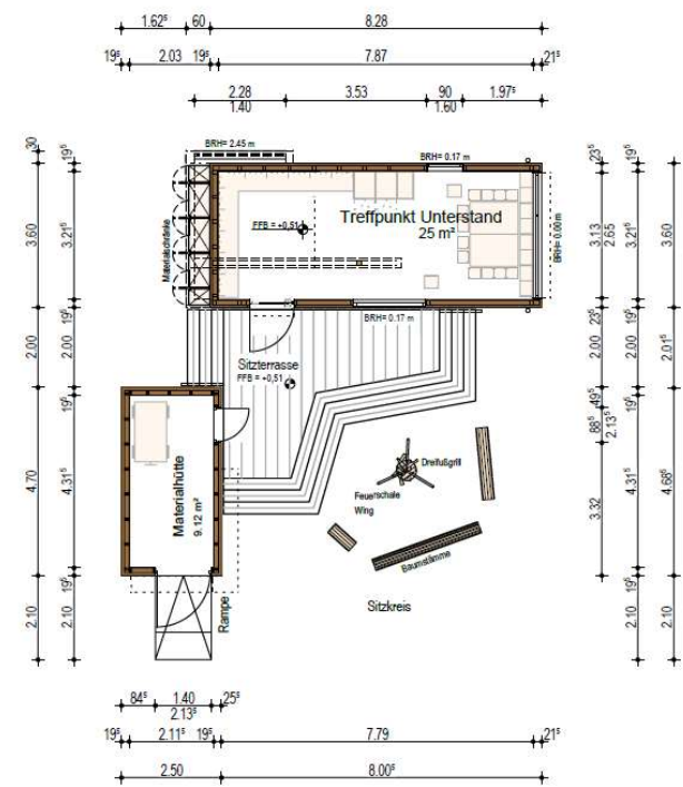
Grundriss Schema Treffpunkt Unterstand + Materialhütte M1/100
