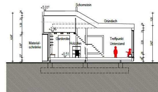
Schnitt M1/100
