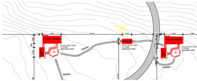
Übersicht Anordnung Hütten M1/500
