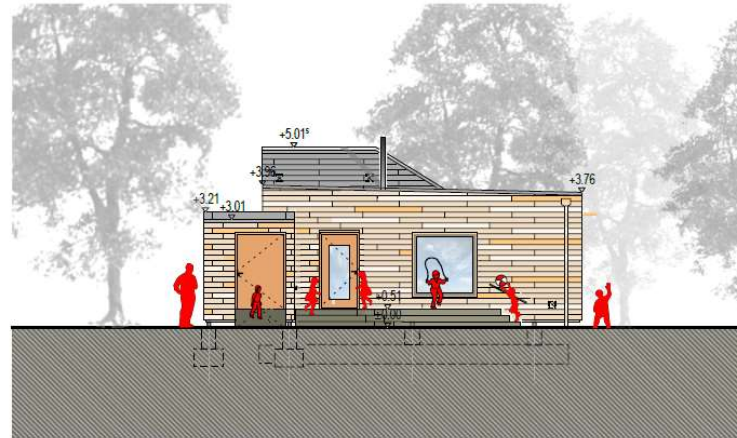
Ansicht Süd M1/100
