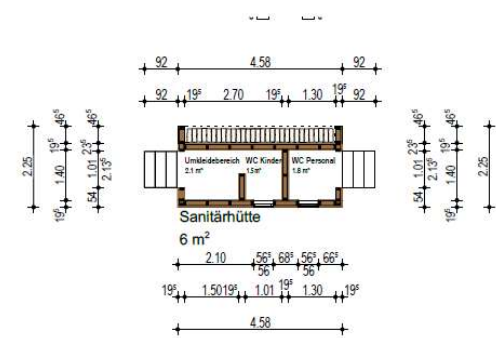
Grundriss Sanitärhütte M1/100
