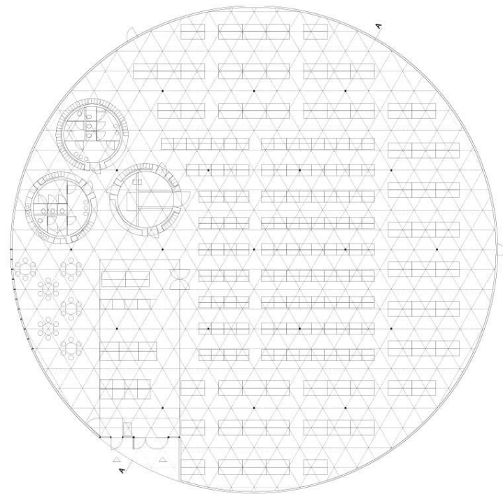
Grundriss M 1:200
