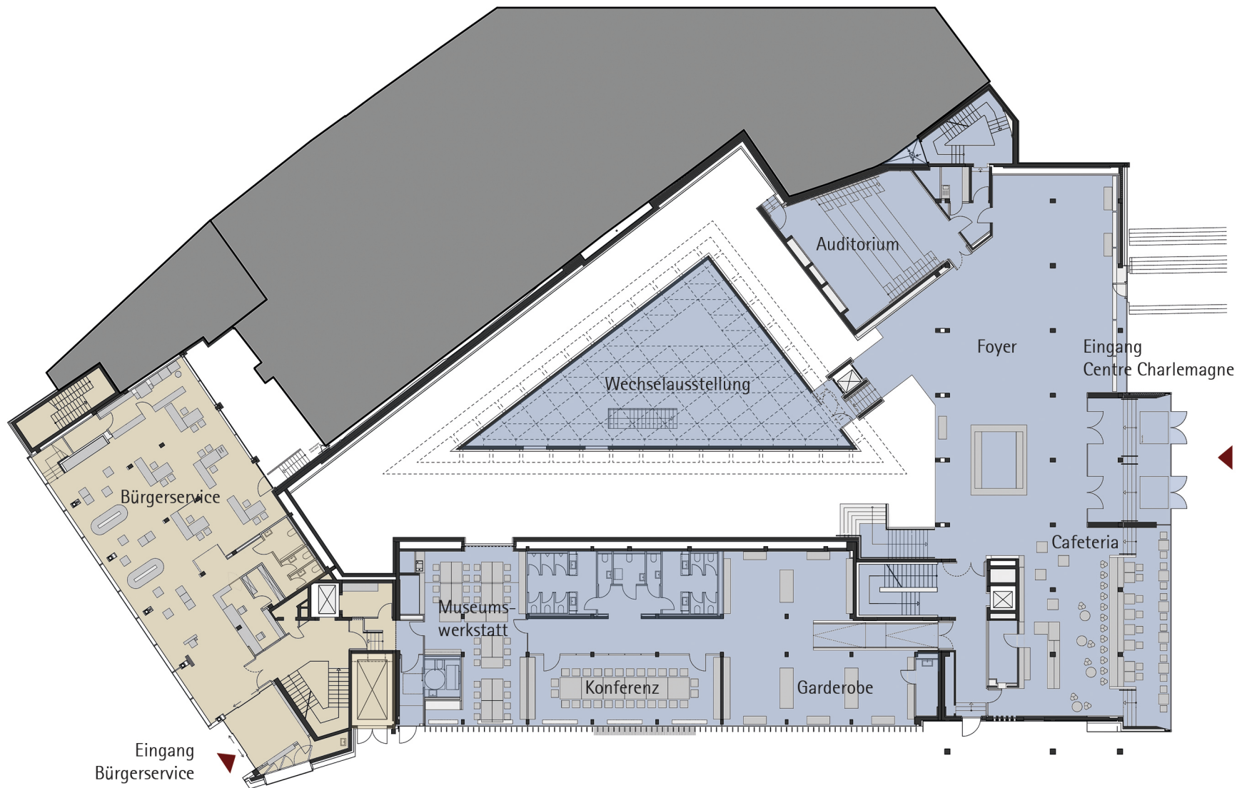
Grundriss EG
