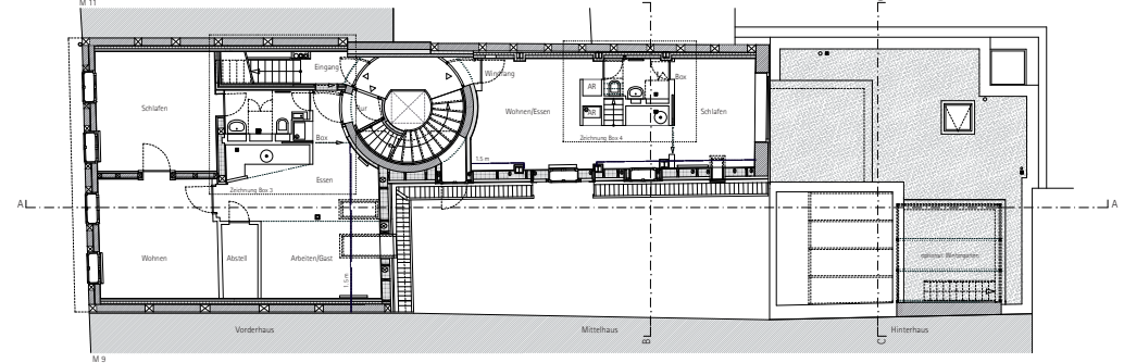
2. Obergeschoss
