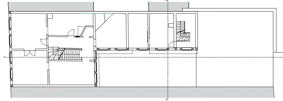
1. Obergeschoss
