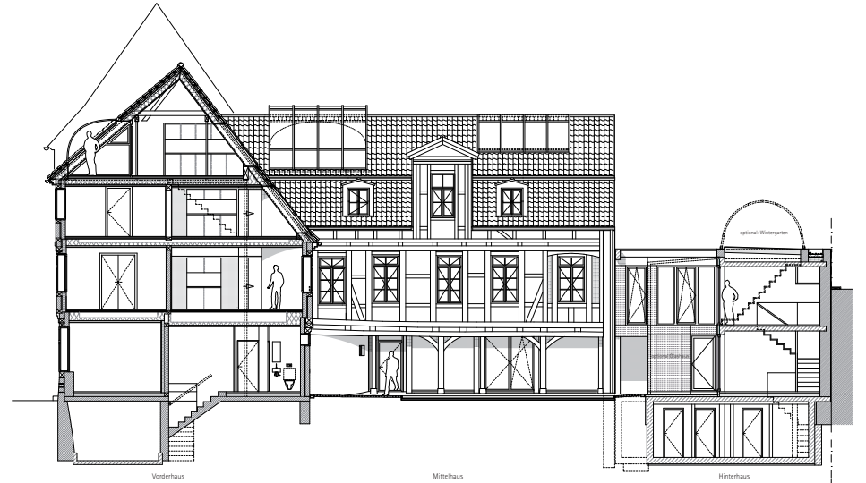
Längsschnitt
