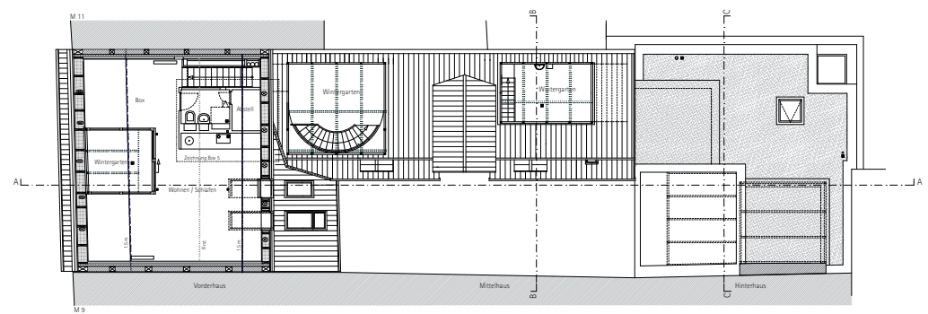
Dachgeschoss
