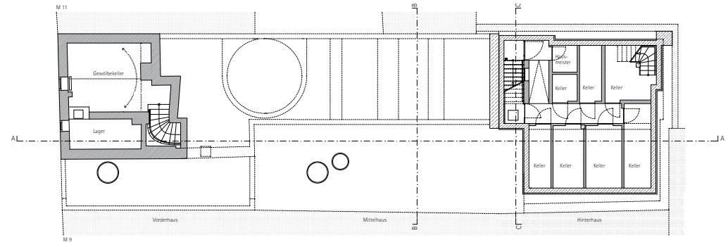
Kellergeschoss
