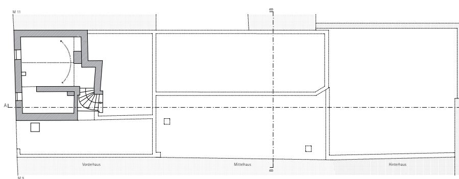
Kellergeschoss
