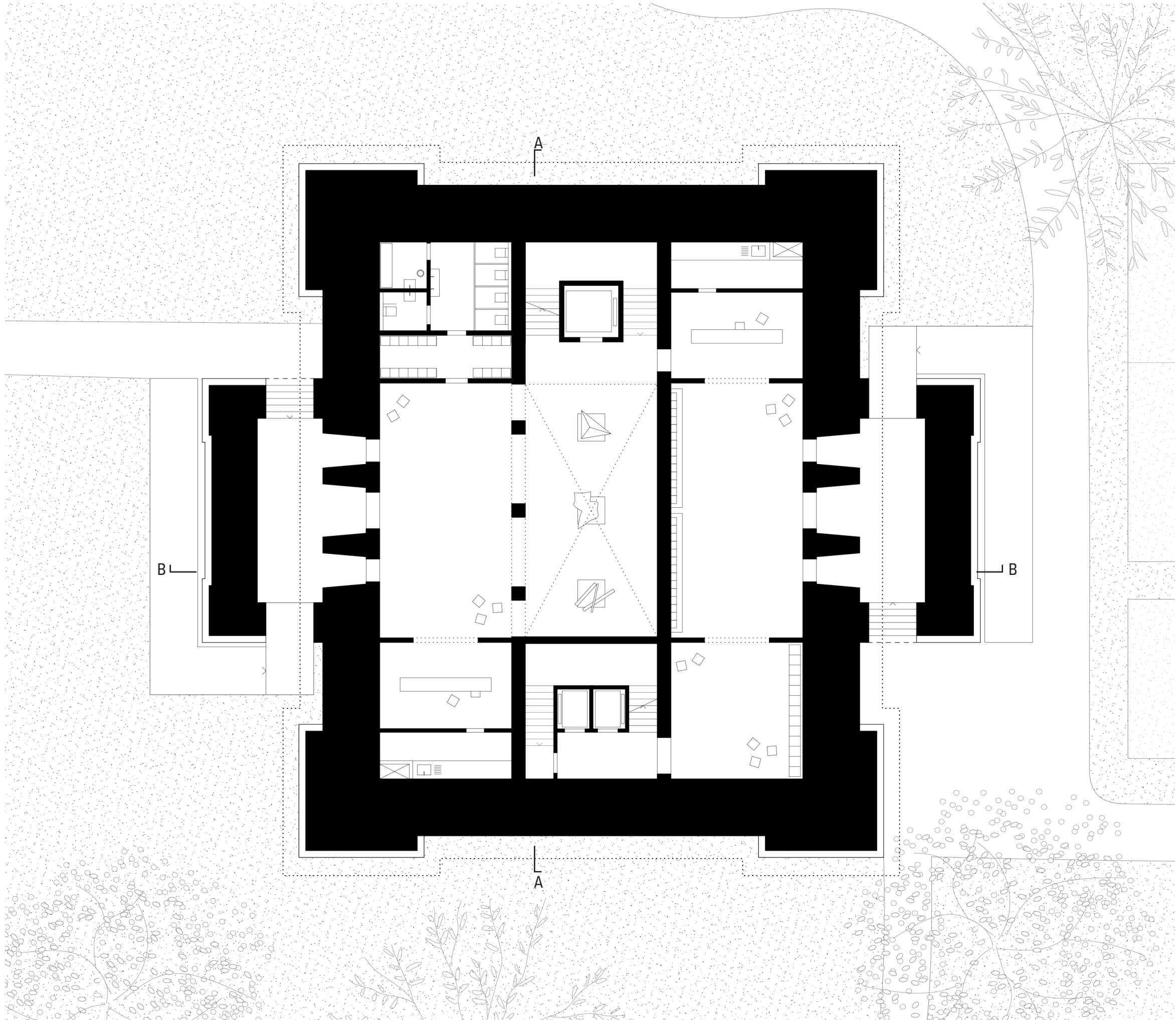
Bunker Erdgeschoss
