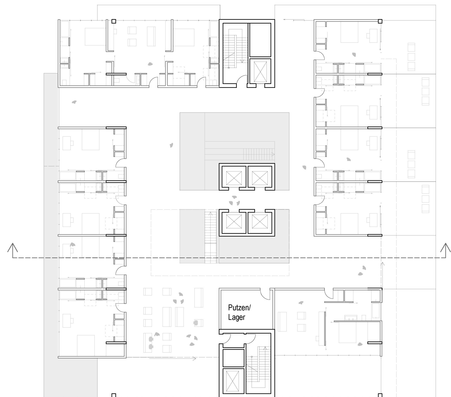
GRUNDRISS NACHBARSCHAFT EBENE 4
