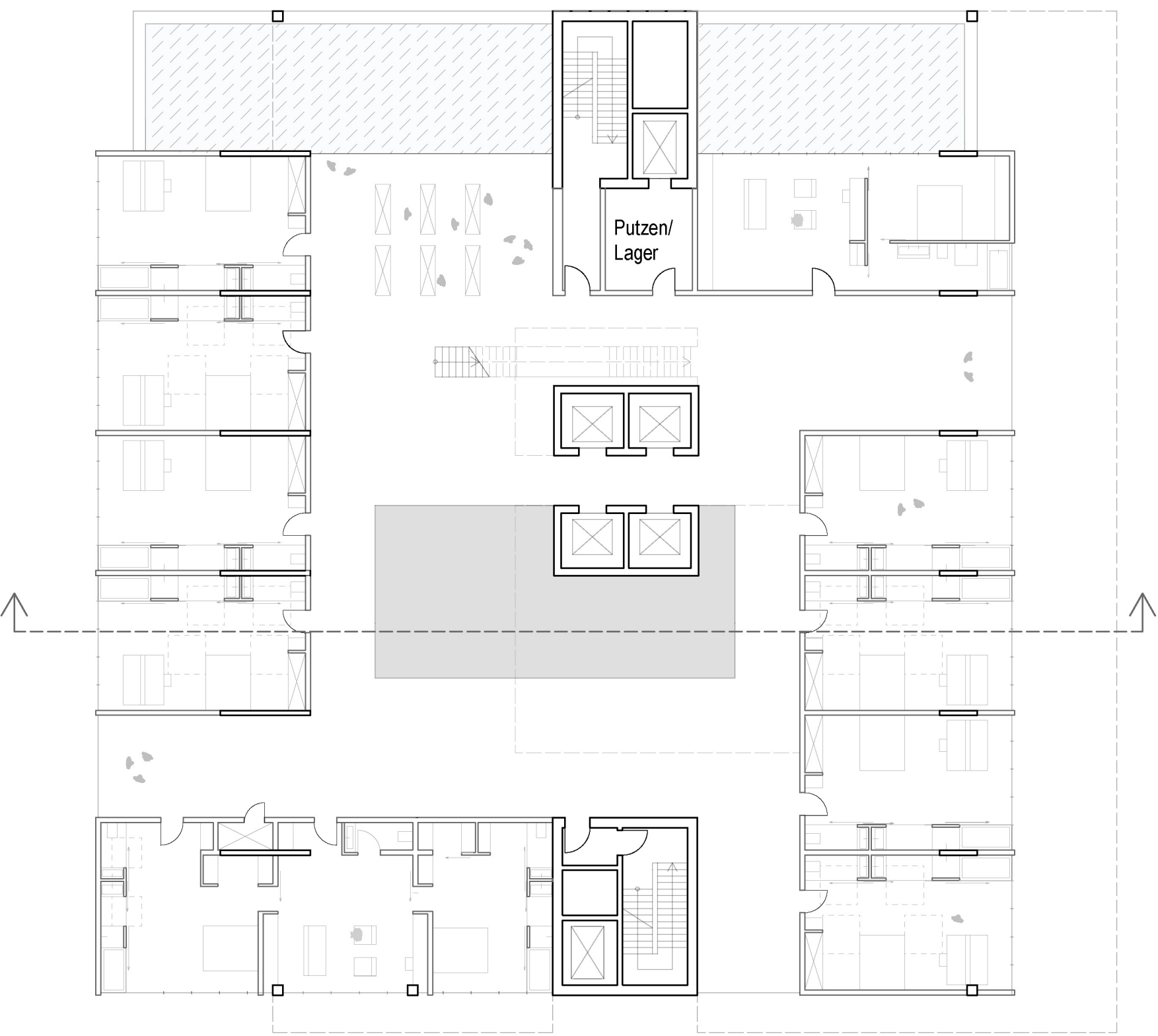
GRUNDRISS NACHBARSCHAFT EBENE 1
