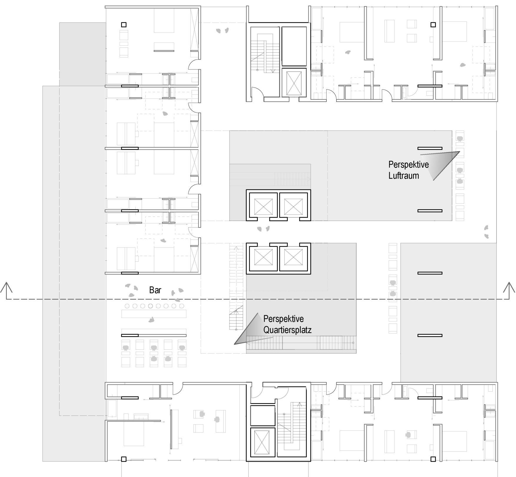
GRUNDRISS NACHBARSCHAFT EBENE 3
