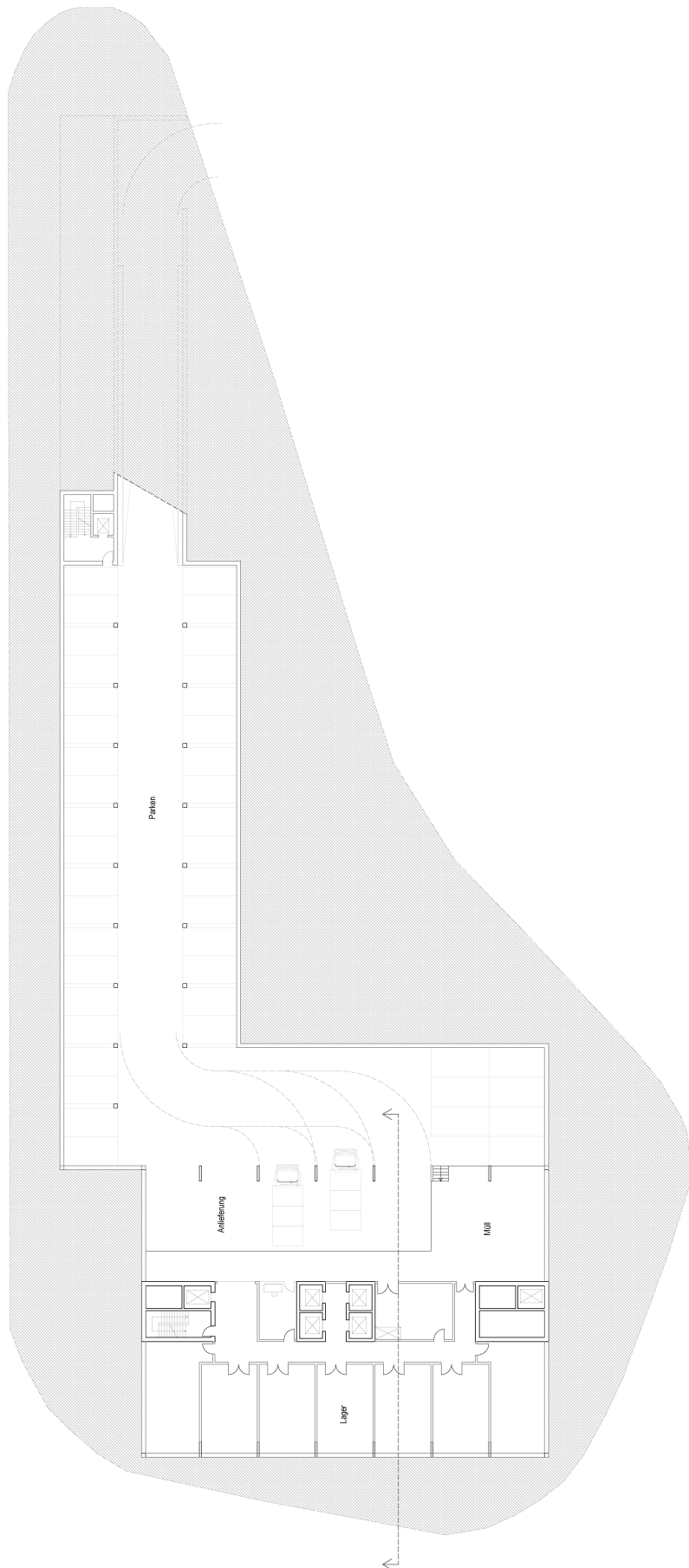
1. UNTERGESCHOSS
