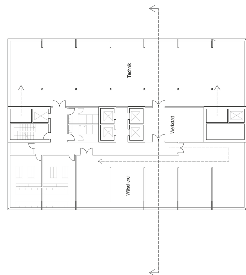
2. UNTERGESCHOSS
