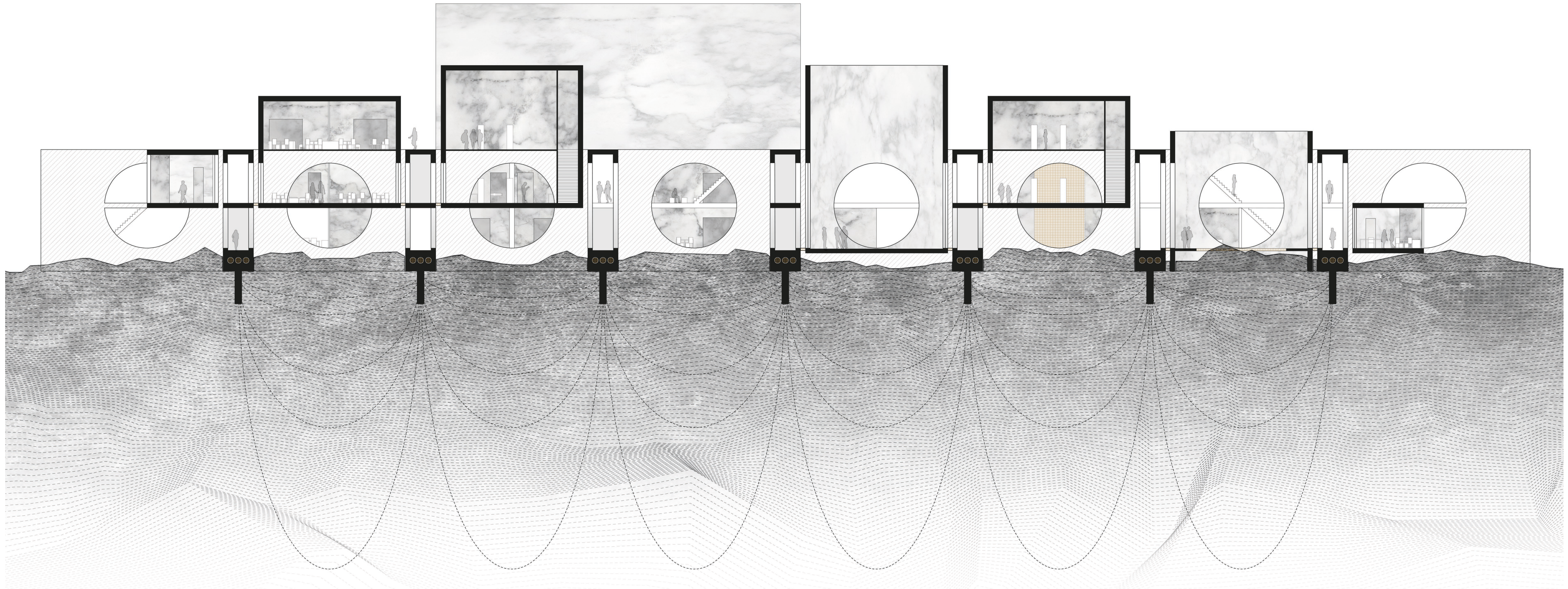
CAMPUS FÜR ANGEWANDTE RESONANZFORSCHUNG | HREPPAR Schnitt | Labor | M 1:200 Regine Ott
