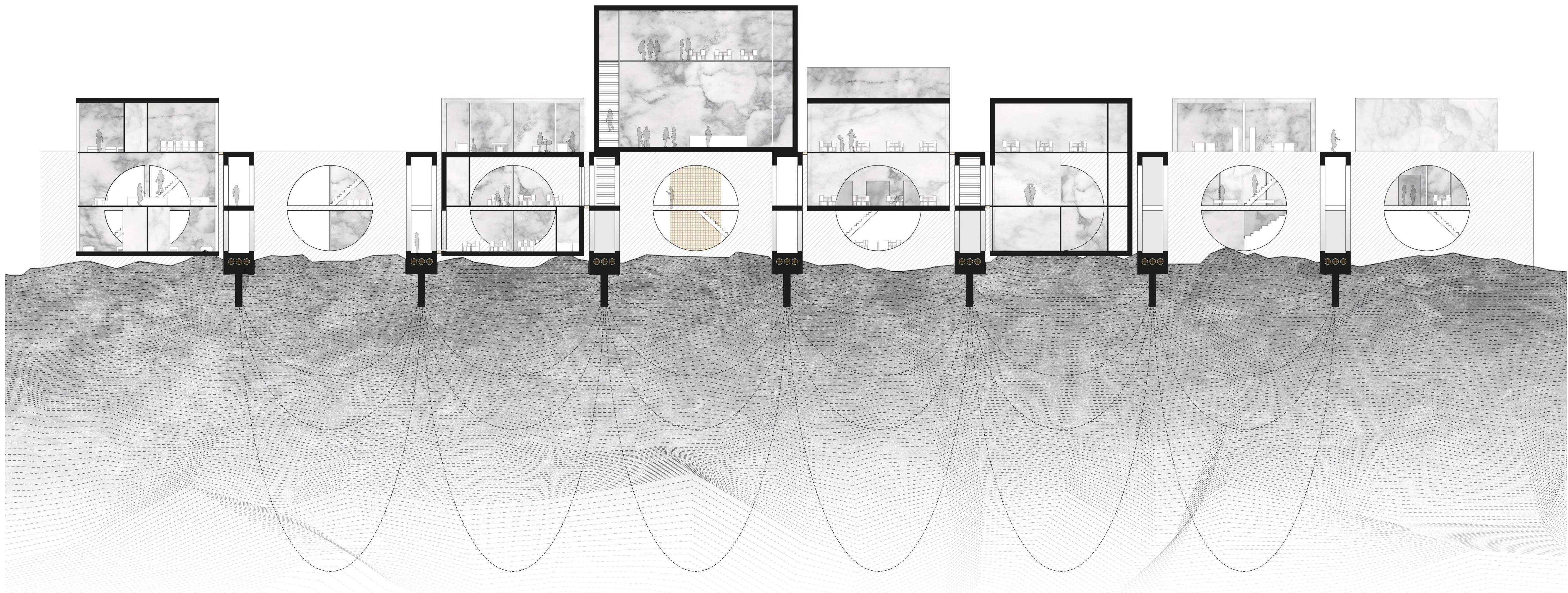
CAMPUS FÜR ANGEWANDTE RESONANZFORSCHUNG | HREPPAR Schnitt | Saal quer | M 1:200 Regine Ott
