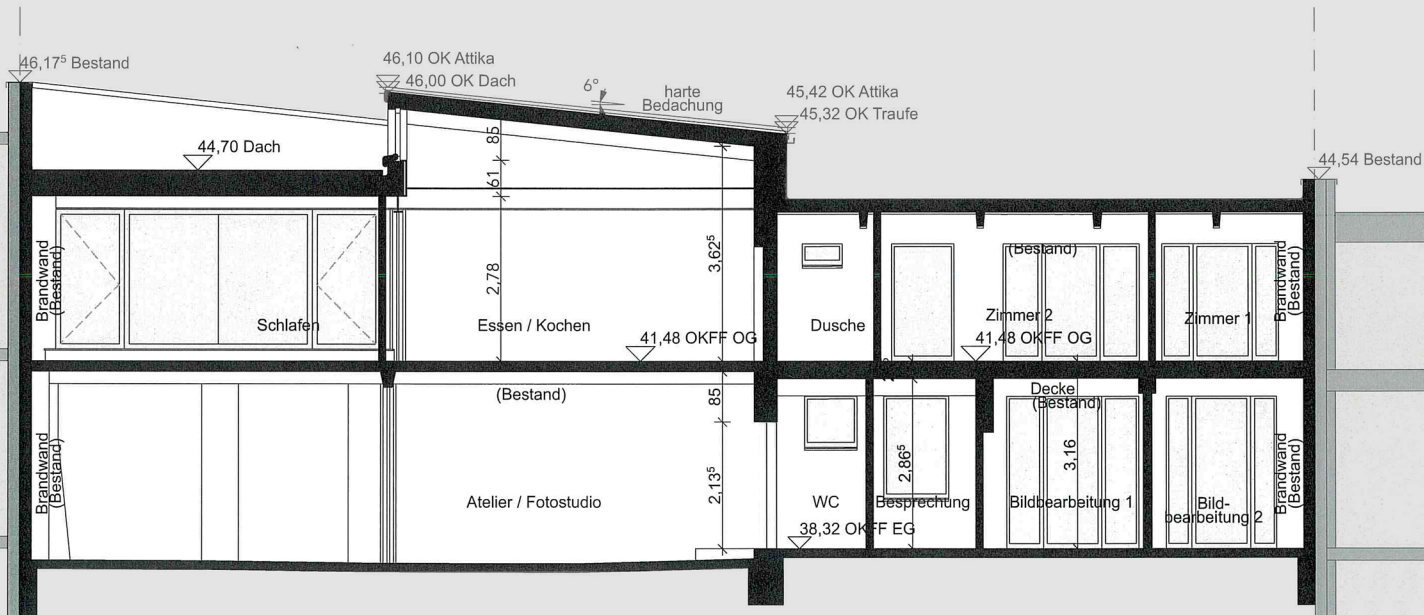
Schnitt B-B
