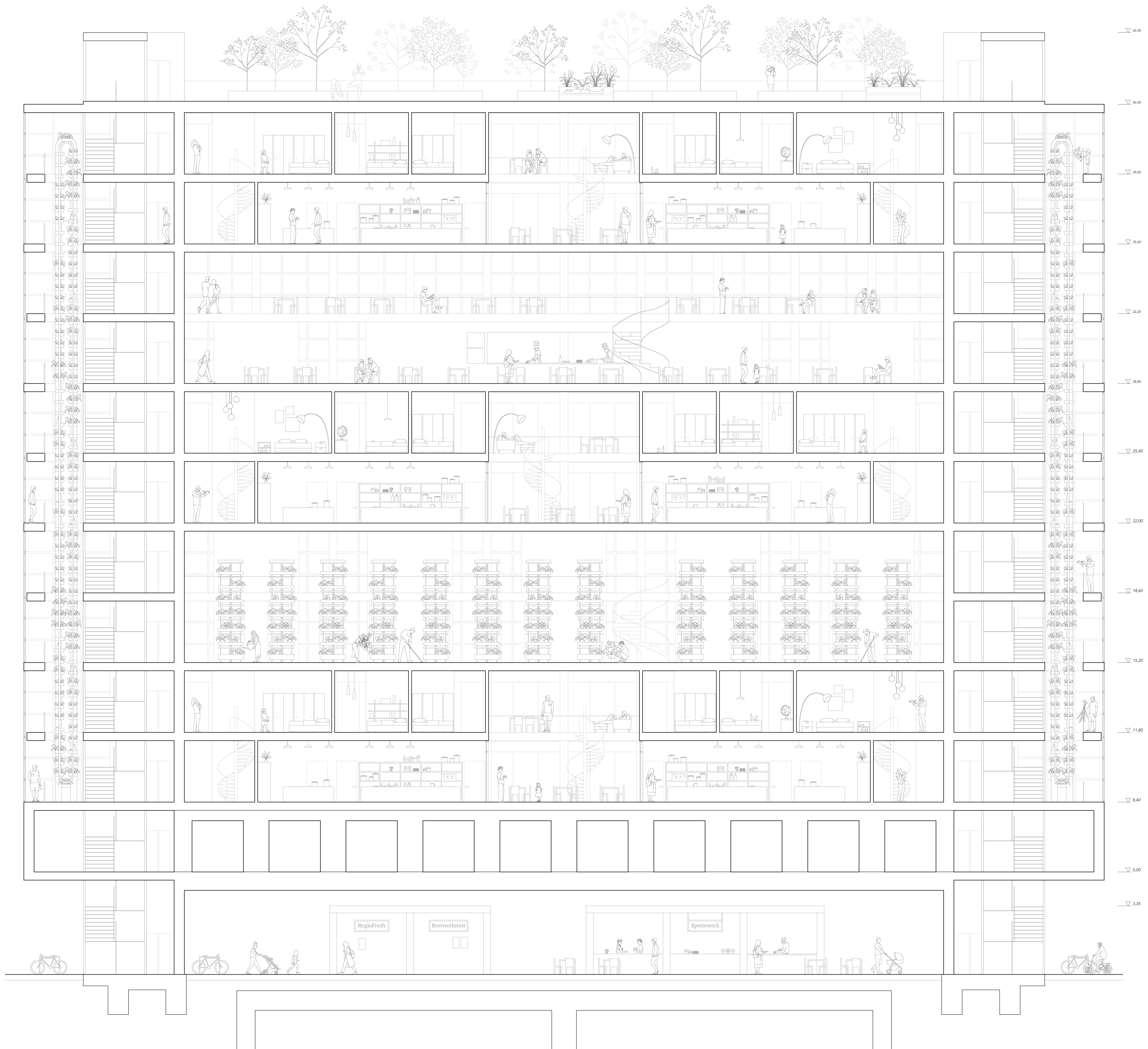
LÄNGSSCHNITT M 1:100
