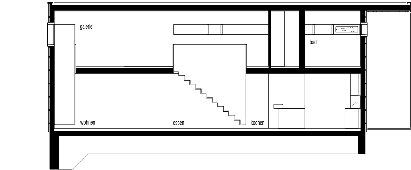
schnitt a
