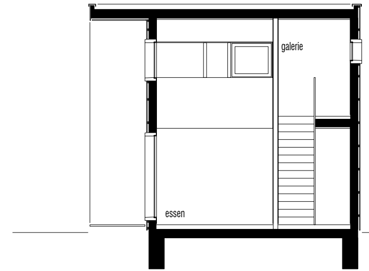
schnitt c
