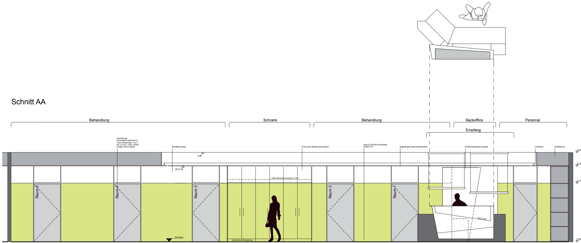
Axonometrie
