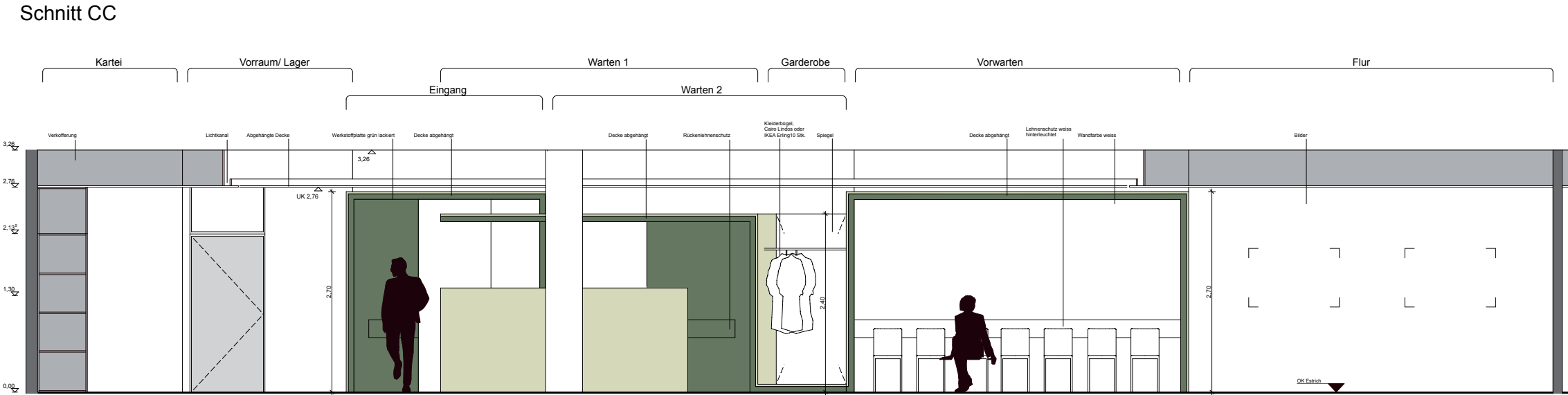
Schnitt CC
