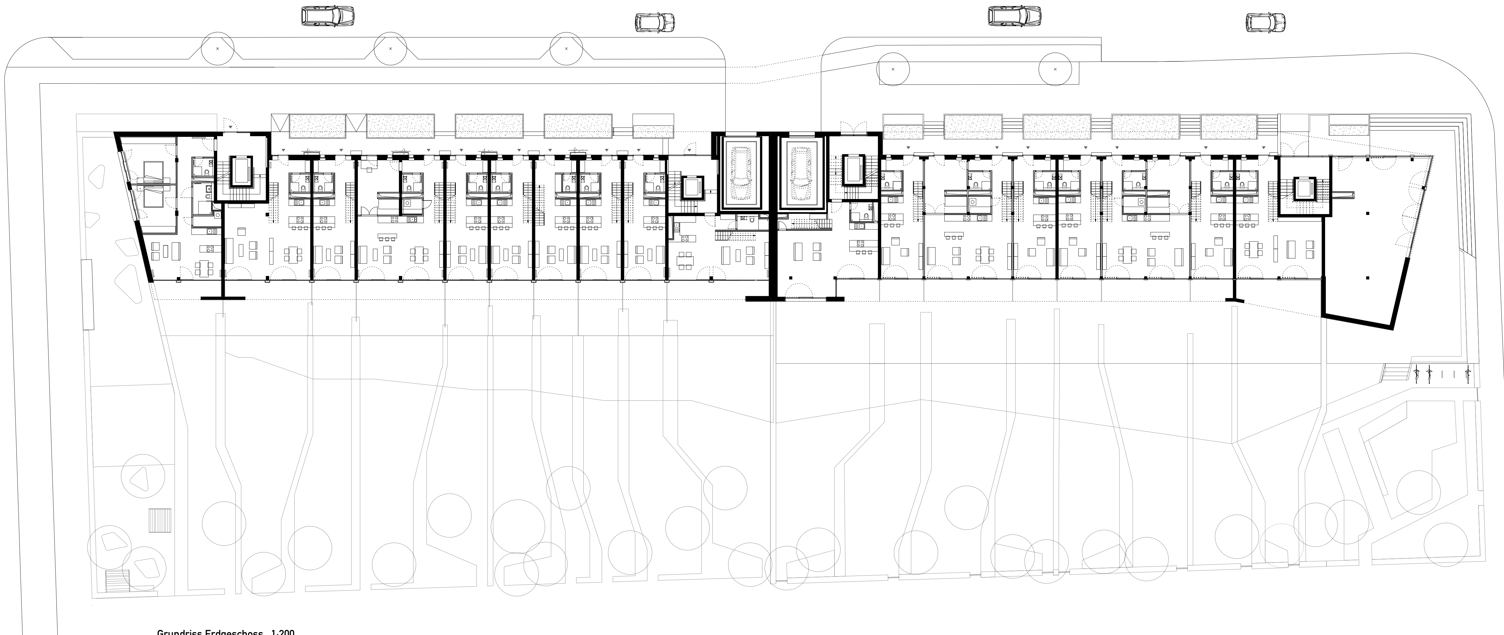
Grundriss Erdgeschoss 1:200
