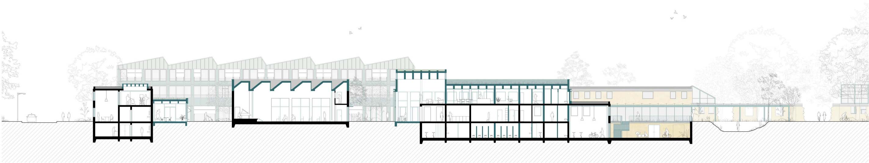
Schnitt A - A Werk - Saal - Forum
