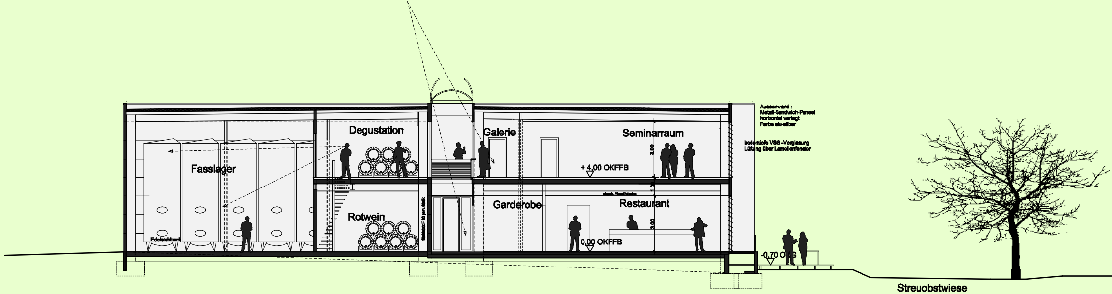
Schnitt B-B
