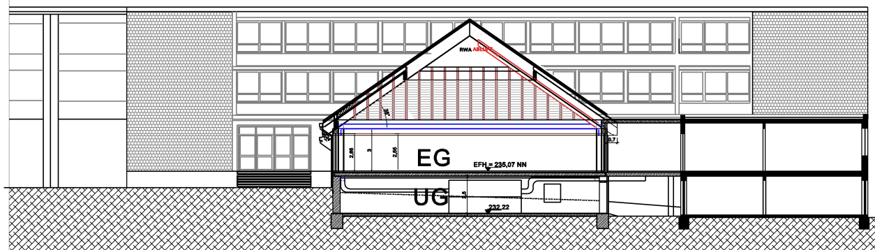
SCHNITT - 2
