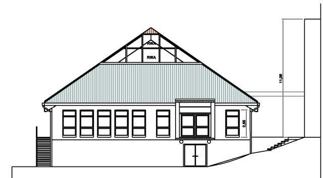
WESTANSICHT
