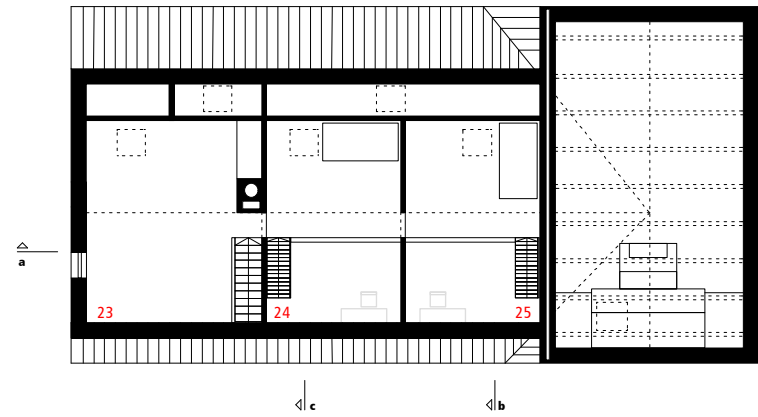
Dachgeschoss
