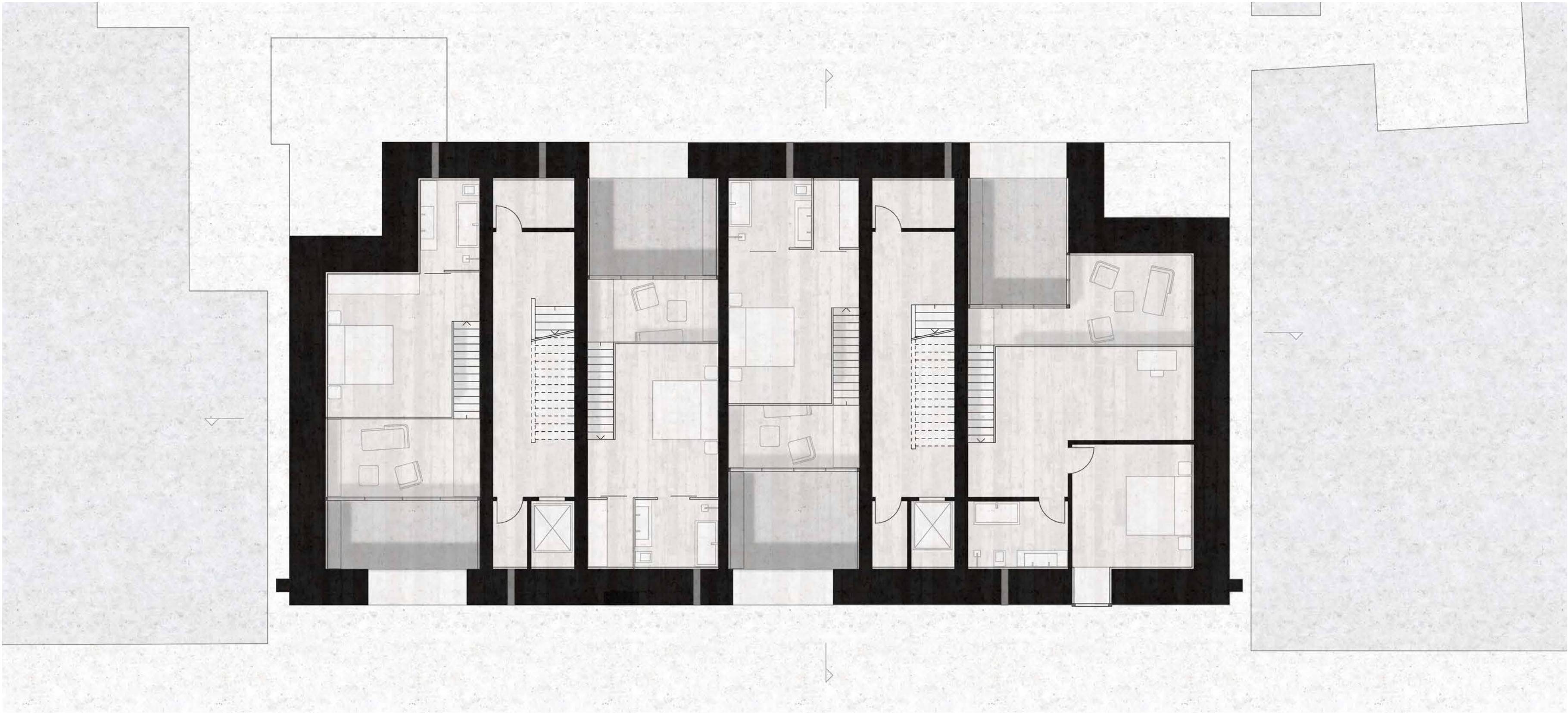
GRUNDRISS 2. OBERGESCHOSS 1:100
