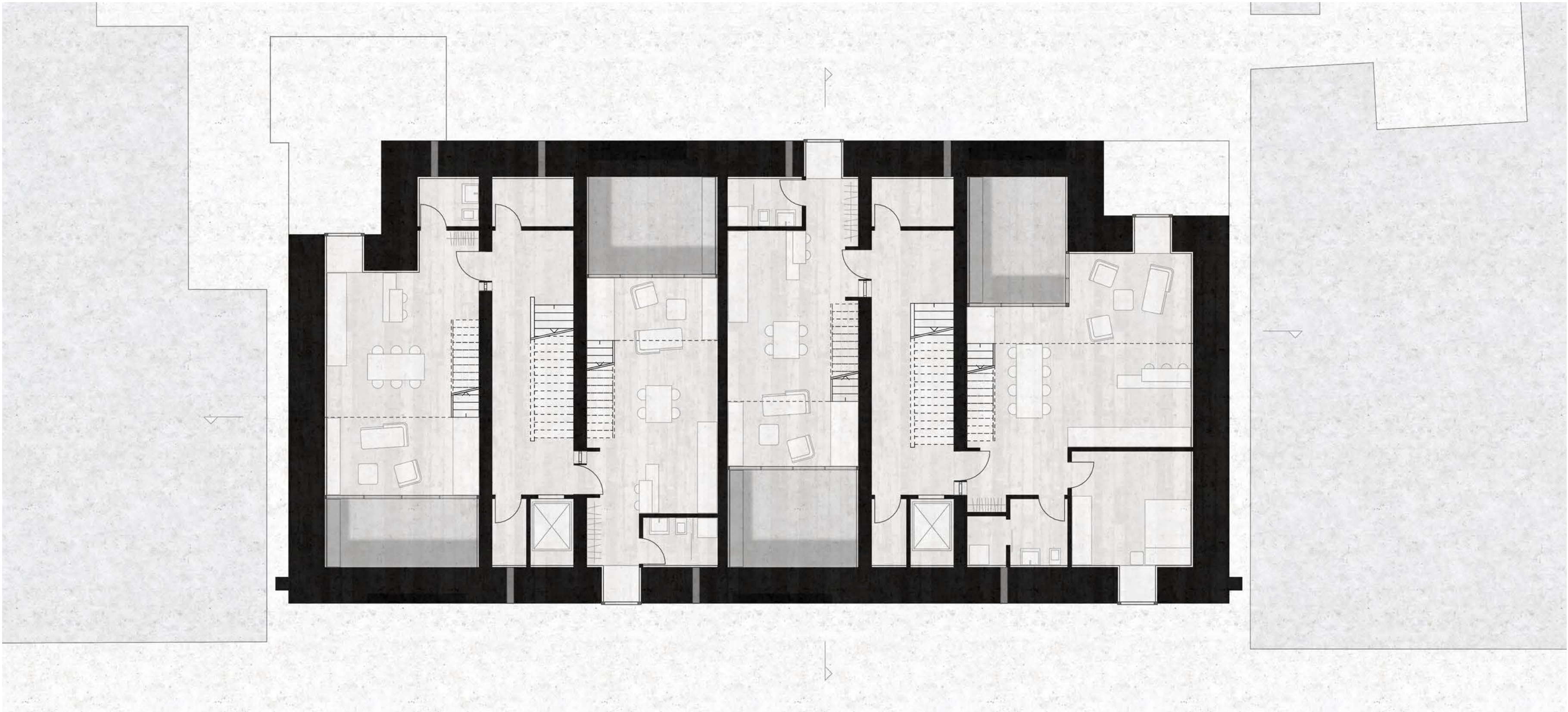
GRUNDRISS 1. OBERGESCHOSS 1:100
