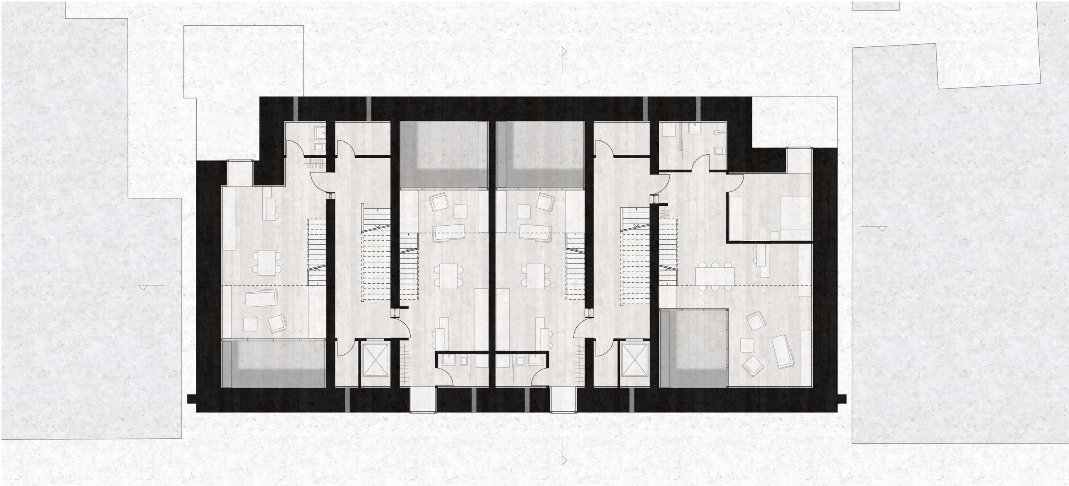
GRUNDRISS 3. OBERGESCHOSS 1:100
