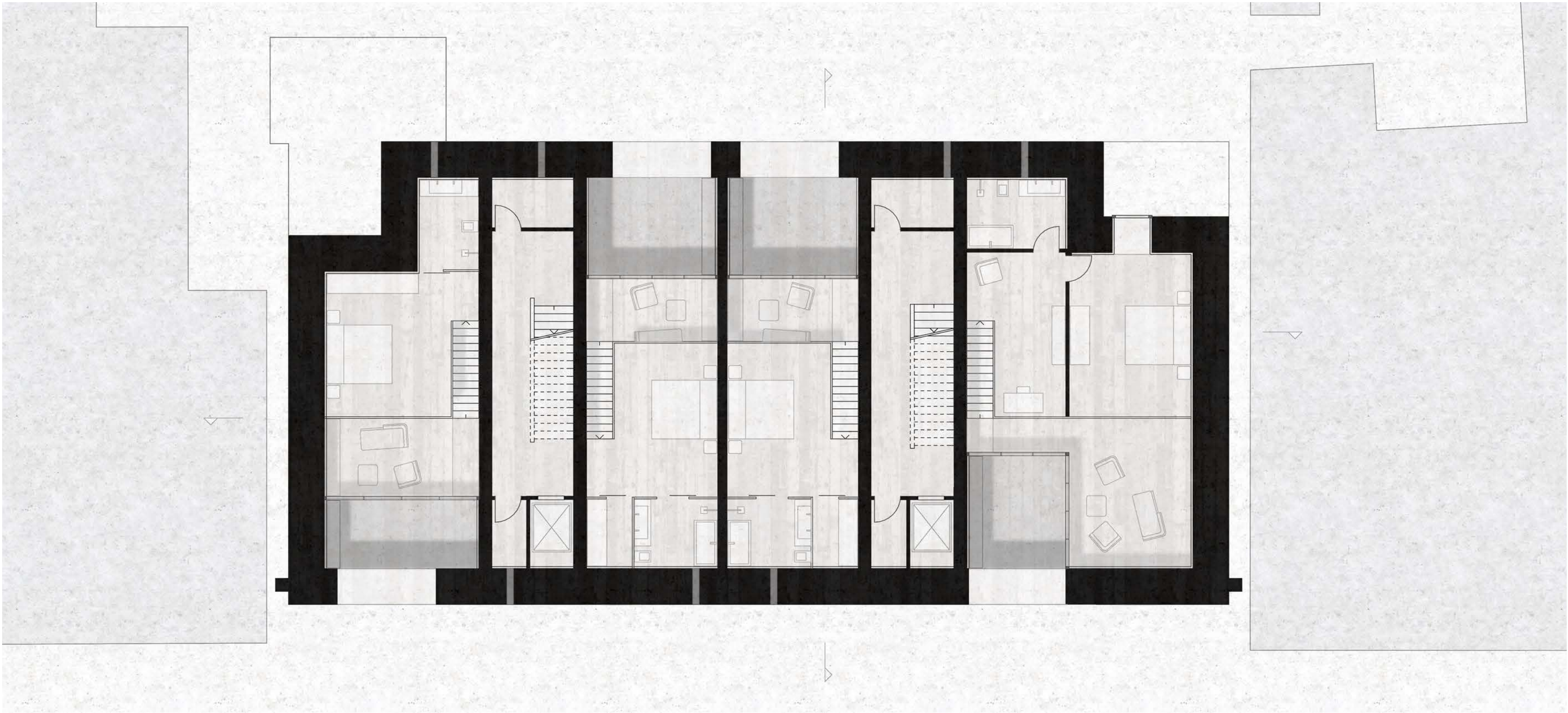
GRUNDRISS 4. OBERGESCHOSS 1:100
