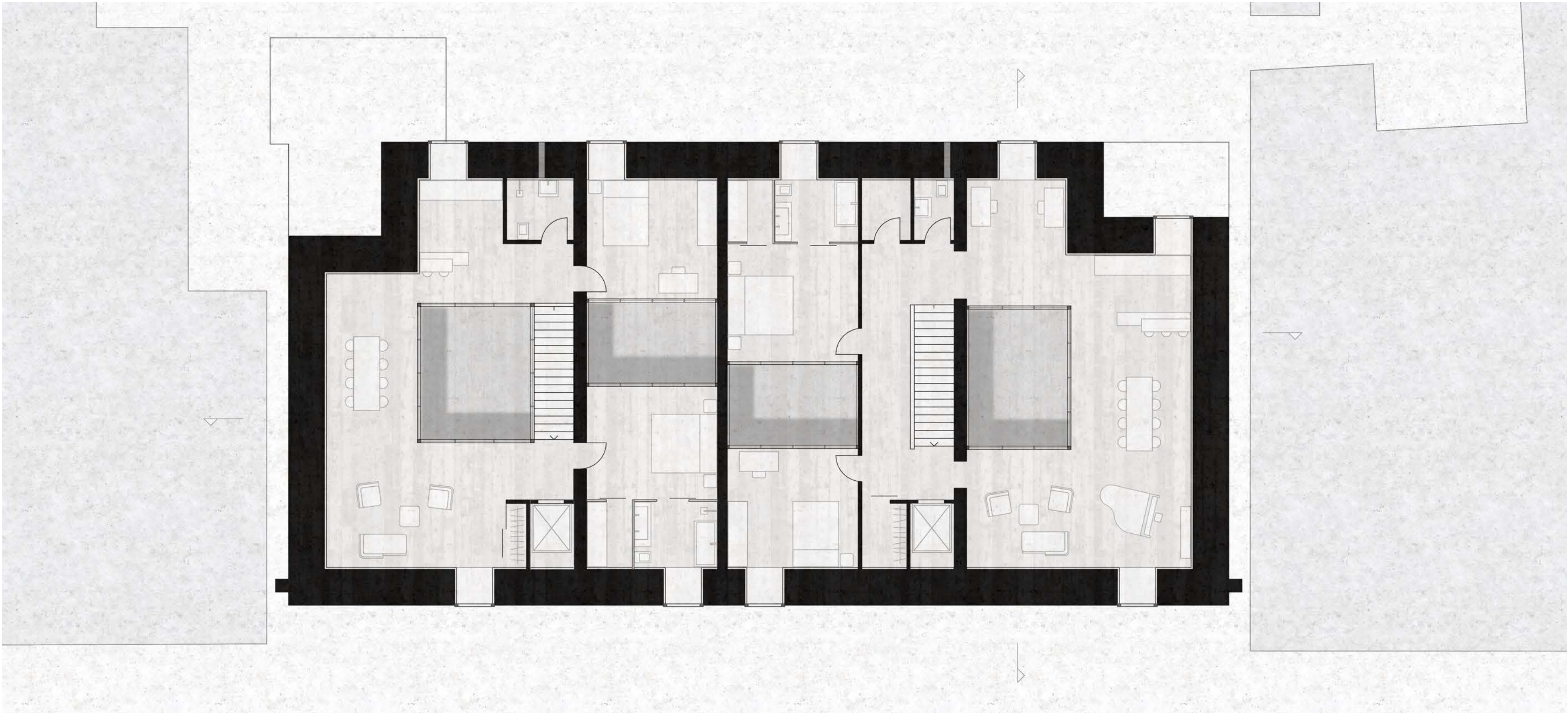
GRUNDRISS 5. OBERGESCHOSS 1:100
