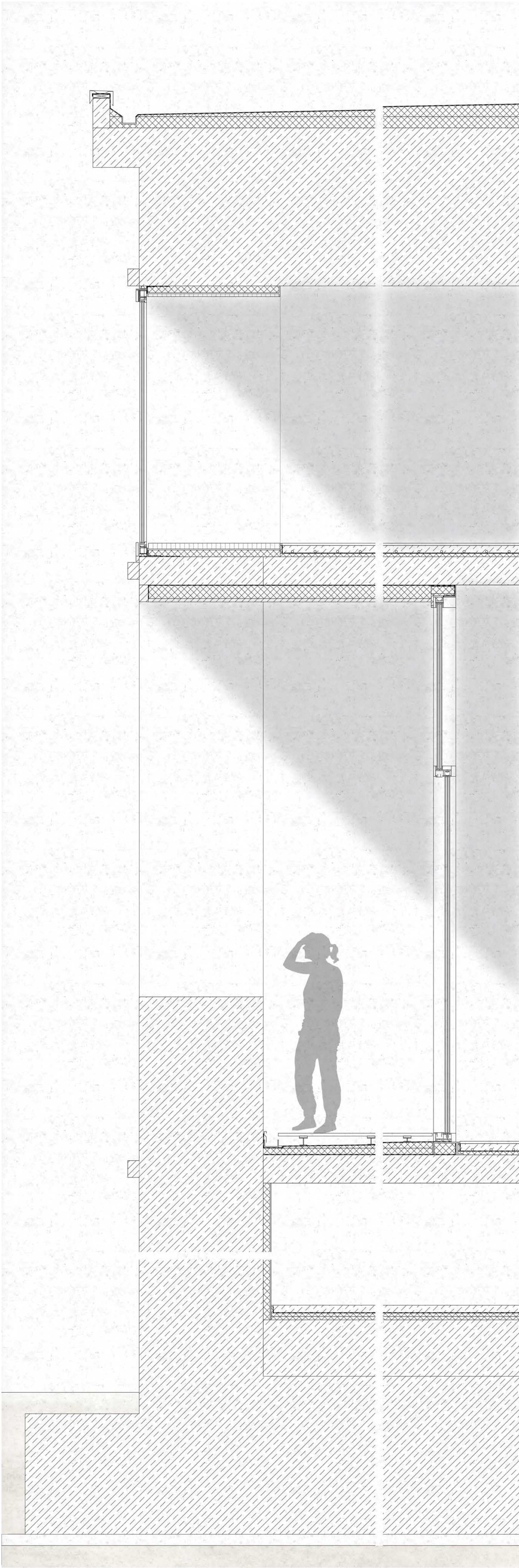
FASSADENSCHNITT 1:20
