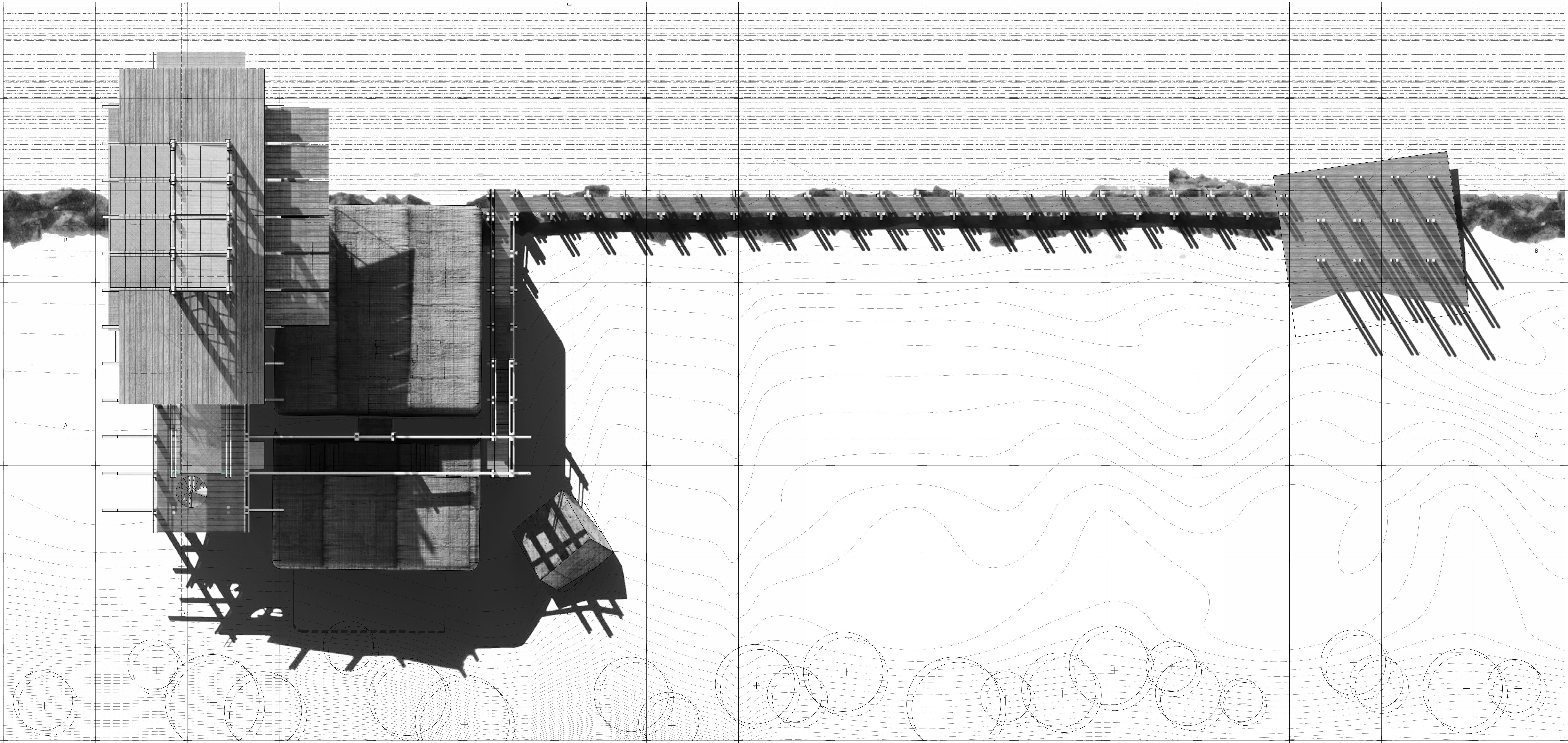
Observatorium Aufsicht M1:100
