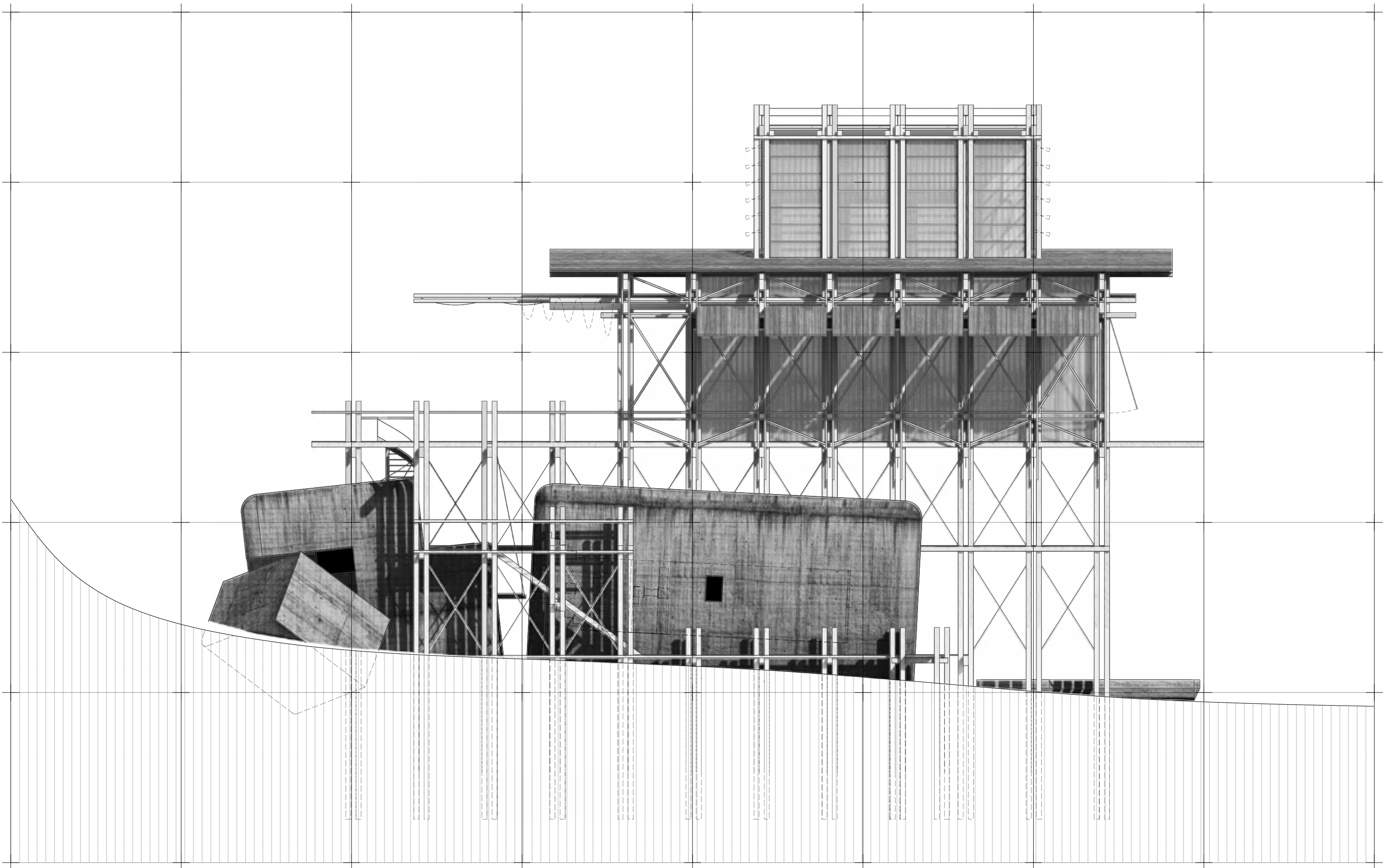
Observatorium Ansicht Ost M1:100
