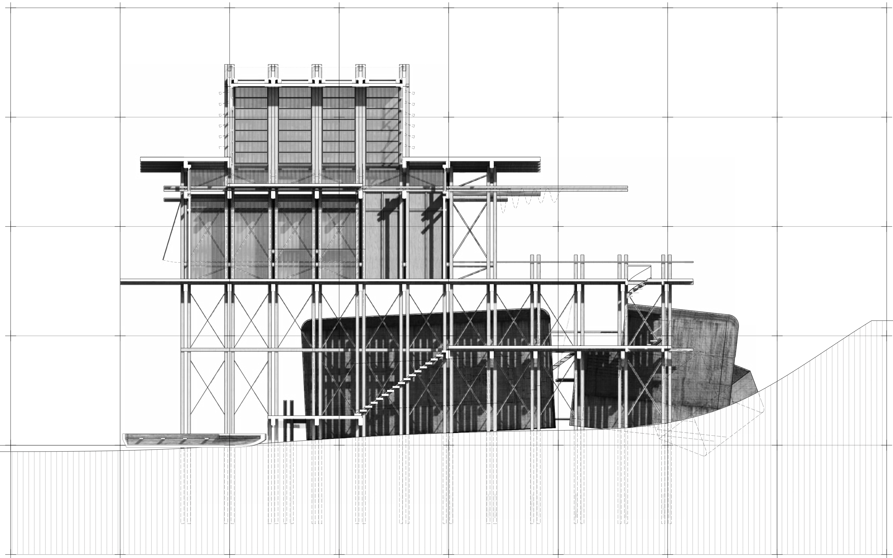
Observatorium Schnitt C-C M1:100
