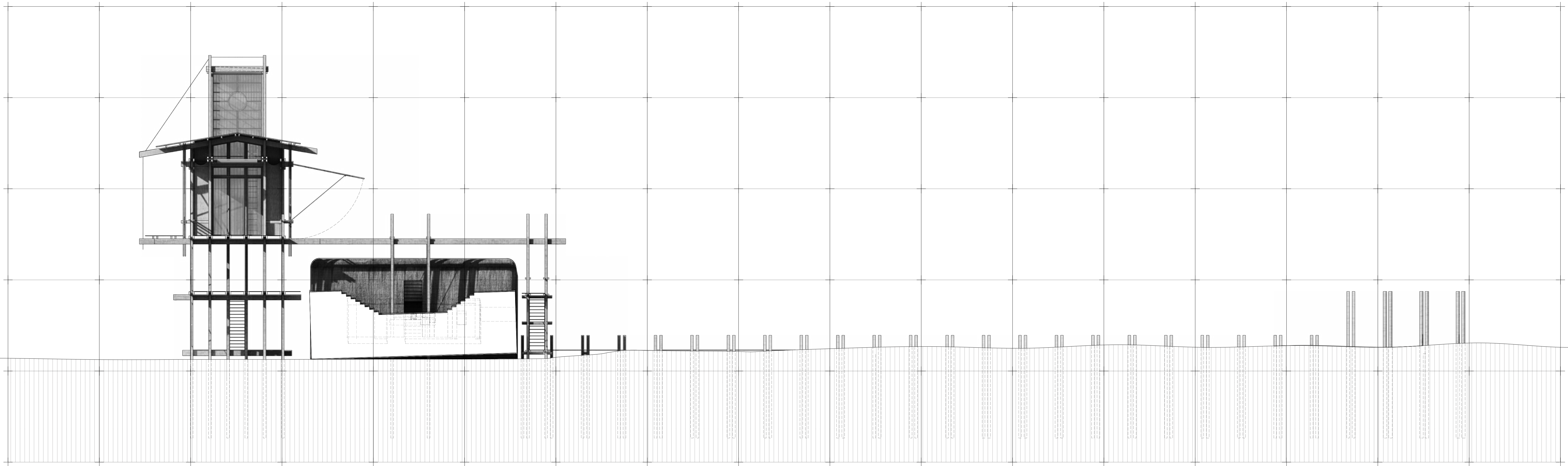
Observatorium Schnitt A-A M1:100
