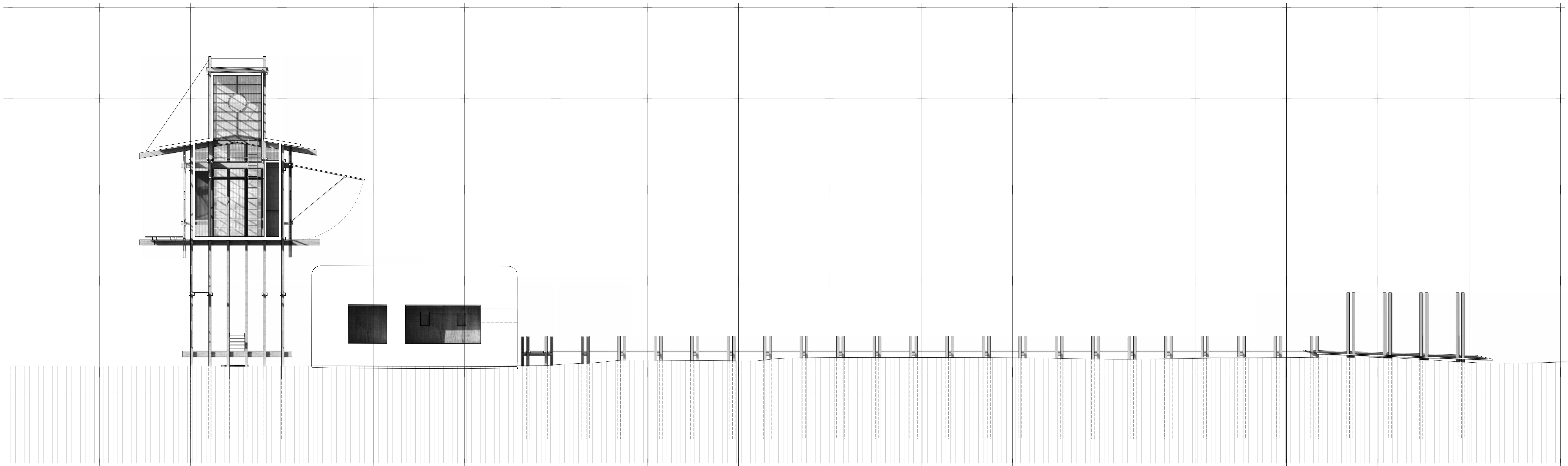
Observatorium Schnitt B-B M1:100
