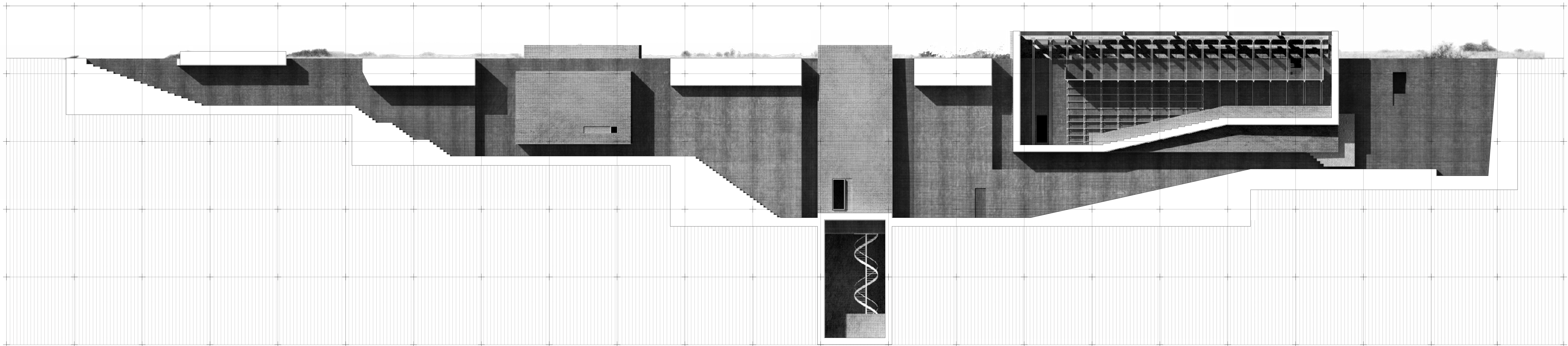
Archiv Schnitt C-C M1:100
