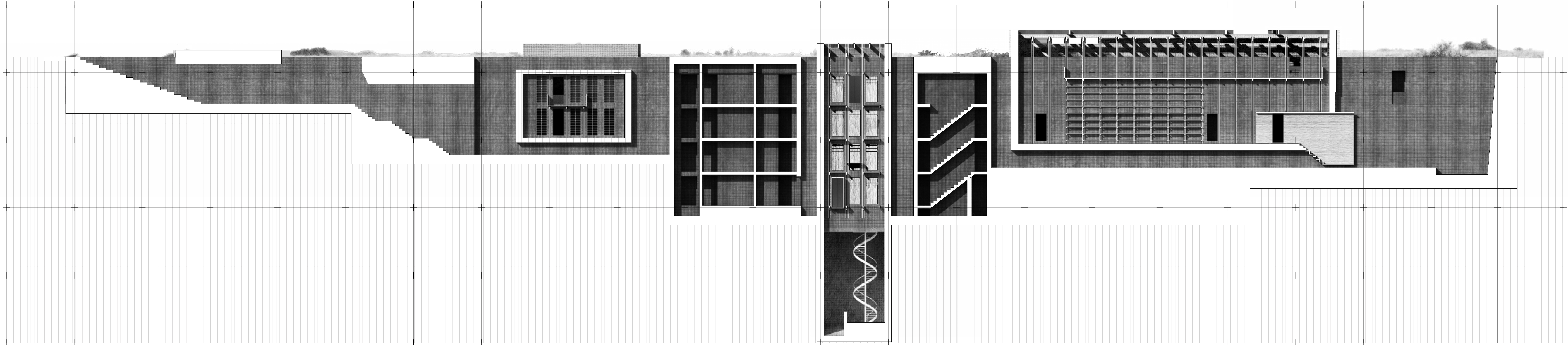
Archiv Schnitt B-B M1:100
