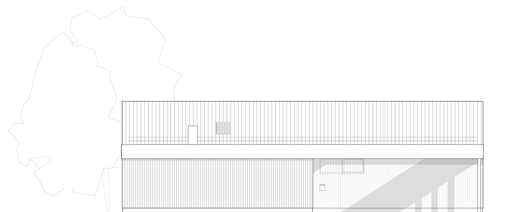
Ansicht Nord
