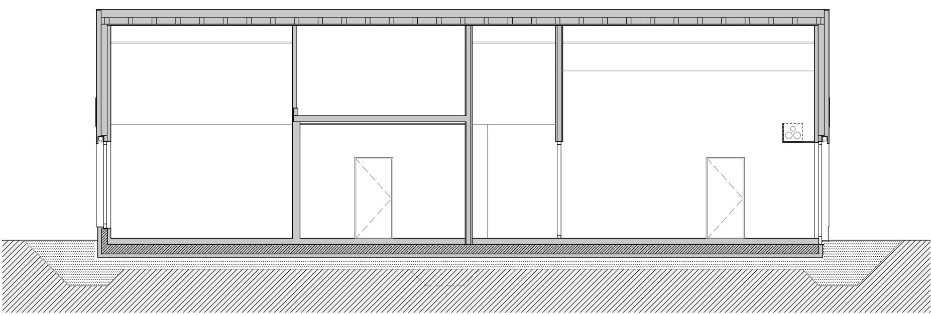
Schnitt S1
