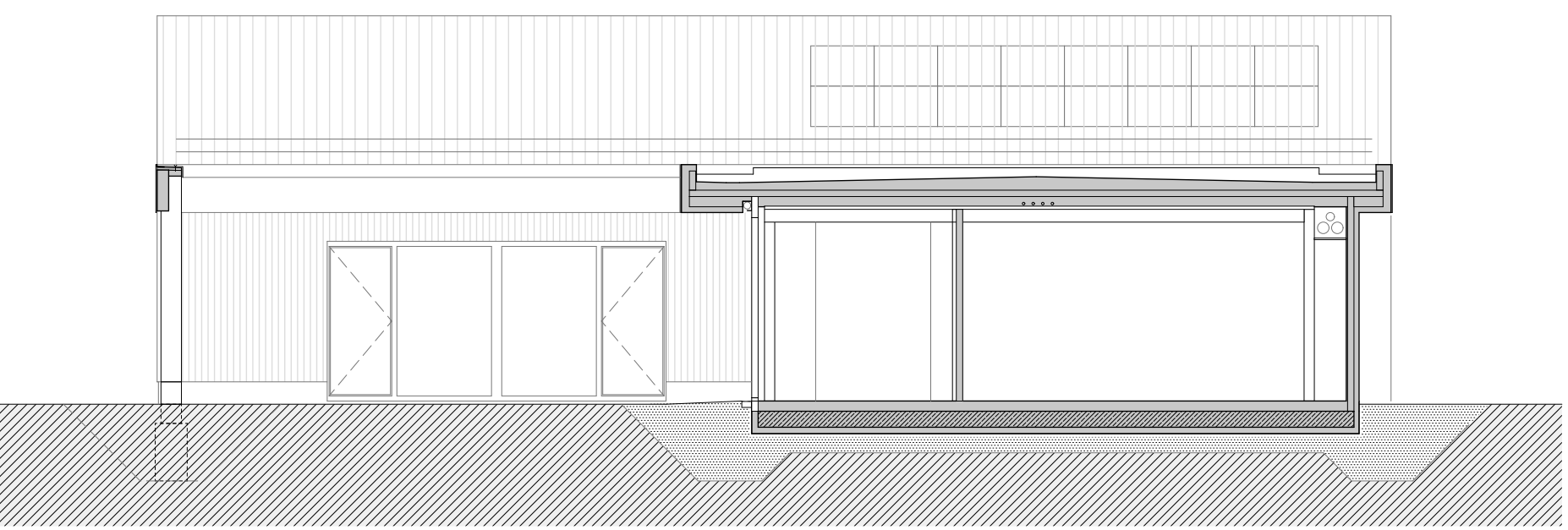
Schnitt S2
