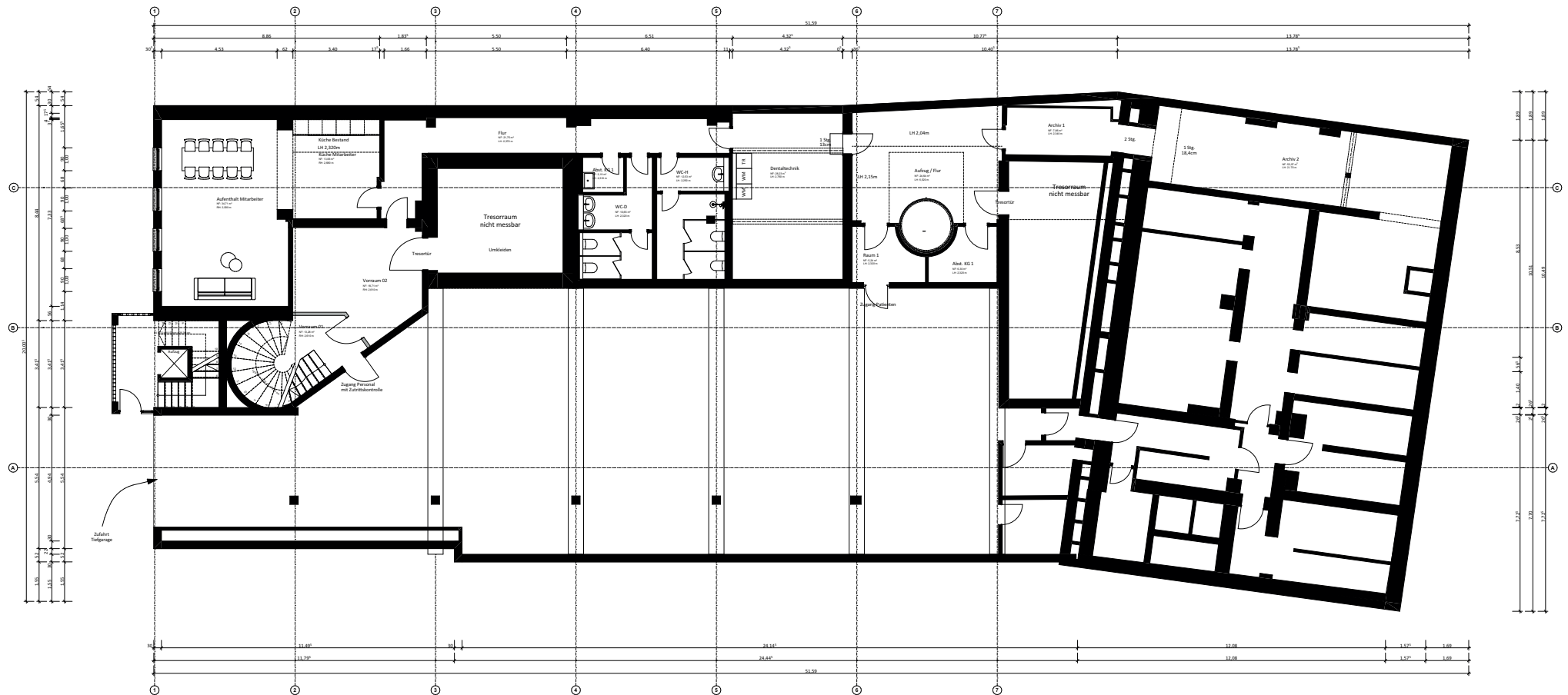
Grundriss | M1:100
