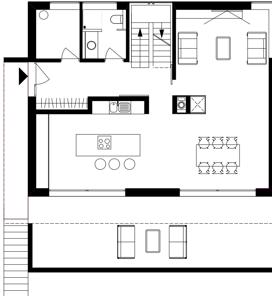
ERDGESCHOSS
