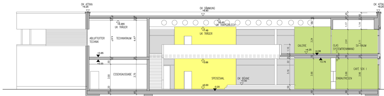
Mensa | Schnitt B-B
